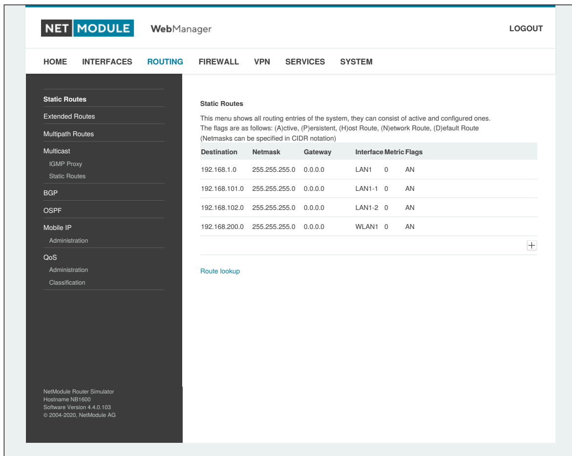
Abbildung 5.24.: Statisches Routing
