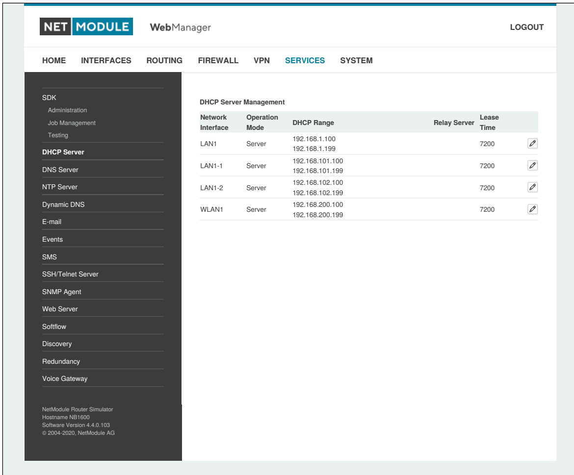
Abbildung 5.42.: DHCP-Server
