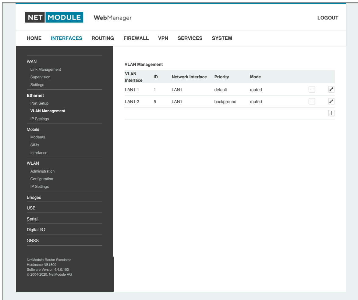
Abbildung 5.8.: VLAN-Verwaltung
