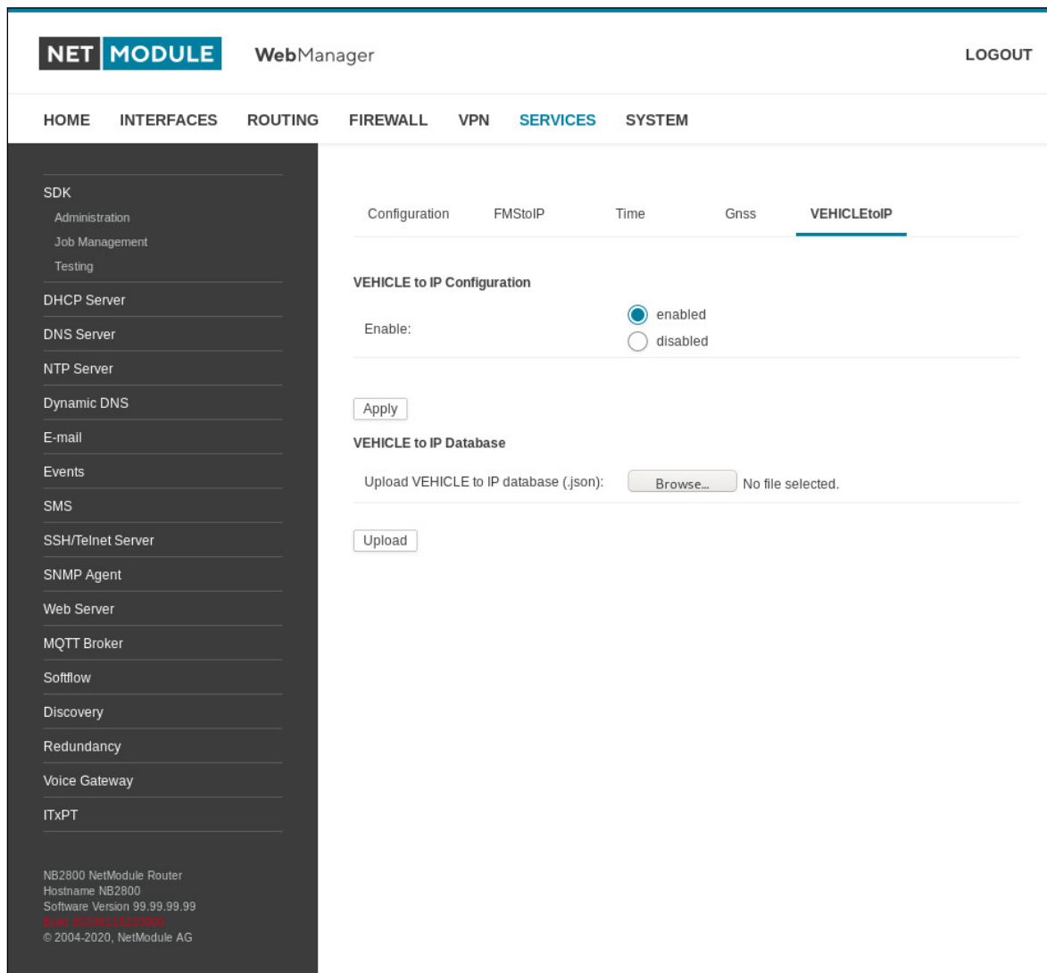
Abbildung 5.58.: ITxPT VEHICLEtoIP
