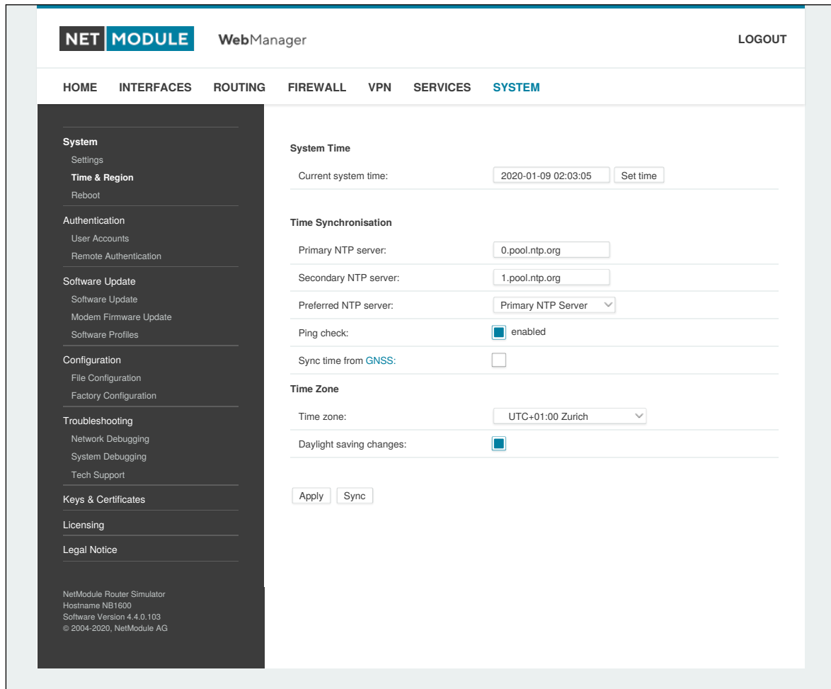
Abbildung 5.63.: Regionseinstellungen
