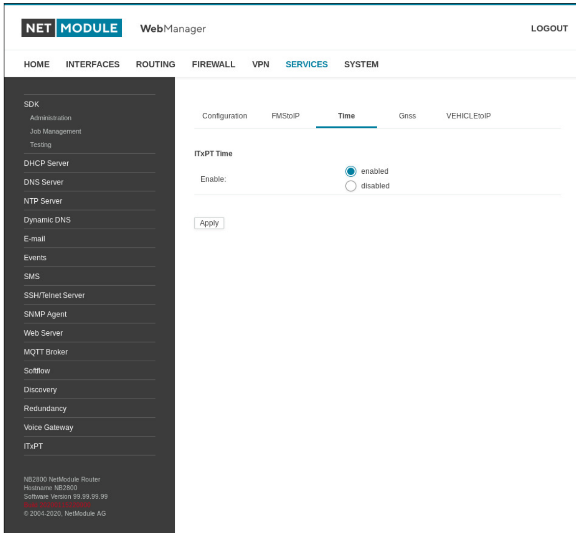
Abbildung 5.56.: ITxPT Time
