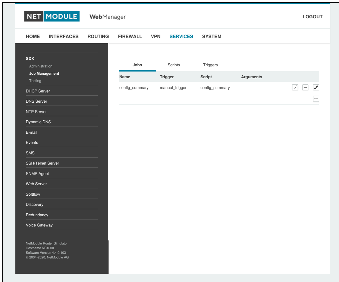
Abbildung 6.42.: SDK-Jobs
