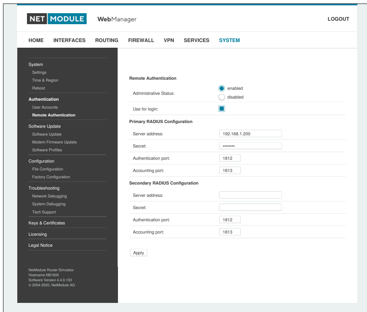
Abbildung 6.69.: Remote-Authentifizierung
