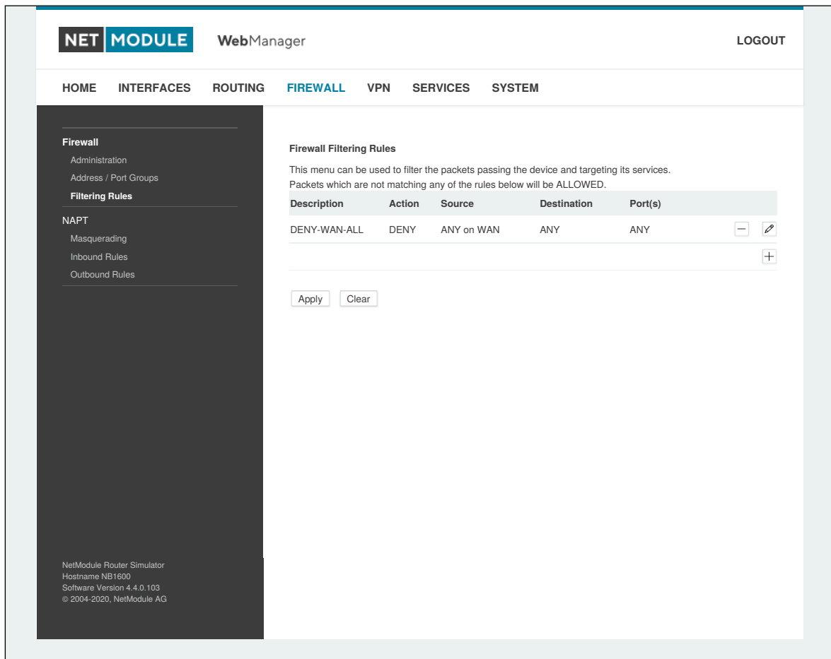
Abbildung 6.30.: Firewall-Regeln
