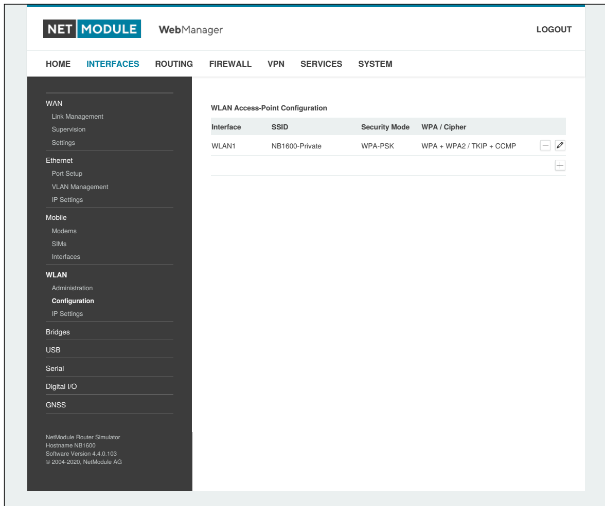
Abbildung 6.19.: WLAN-Konfiguration
