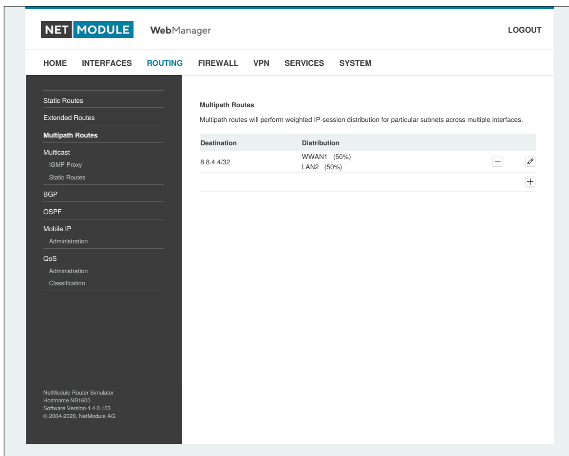
Abbildung 6.26.: Multipath-Routing
