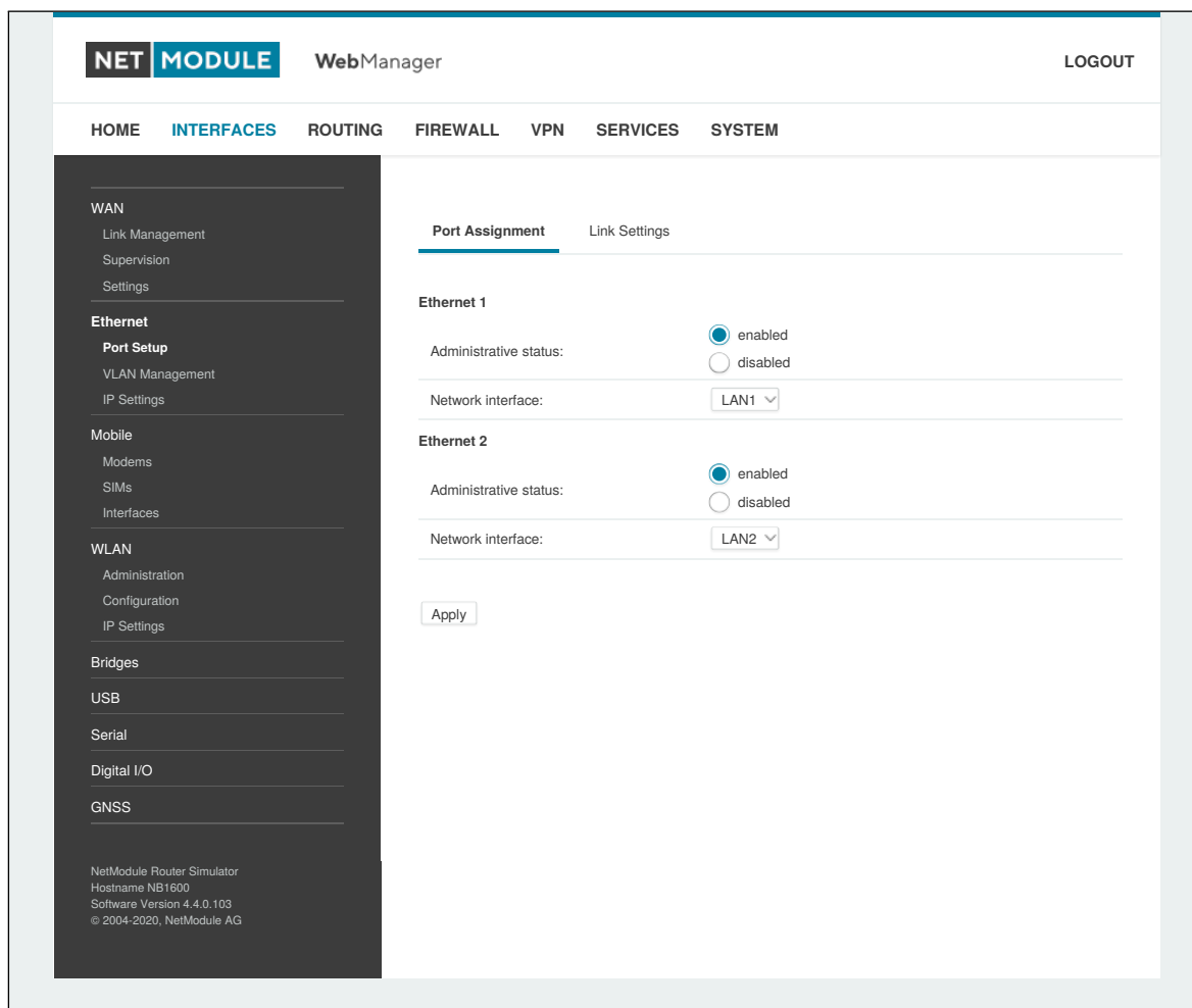
Abbildung 6.6.: Ethernet-Anschlüsse
