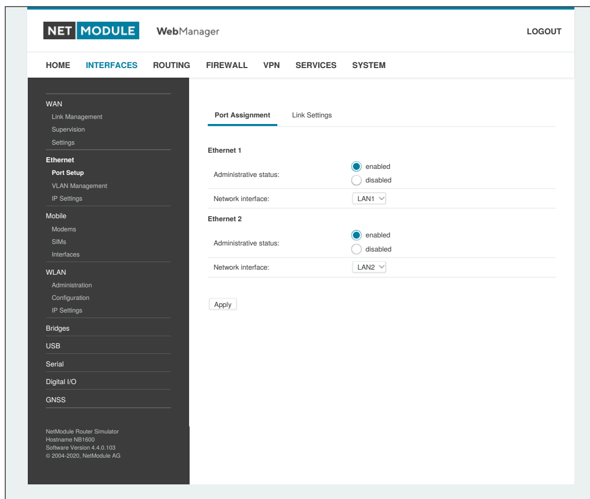
Abbildung 6.5.: Ethernet-Anschlüsse
