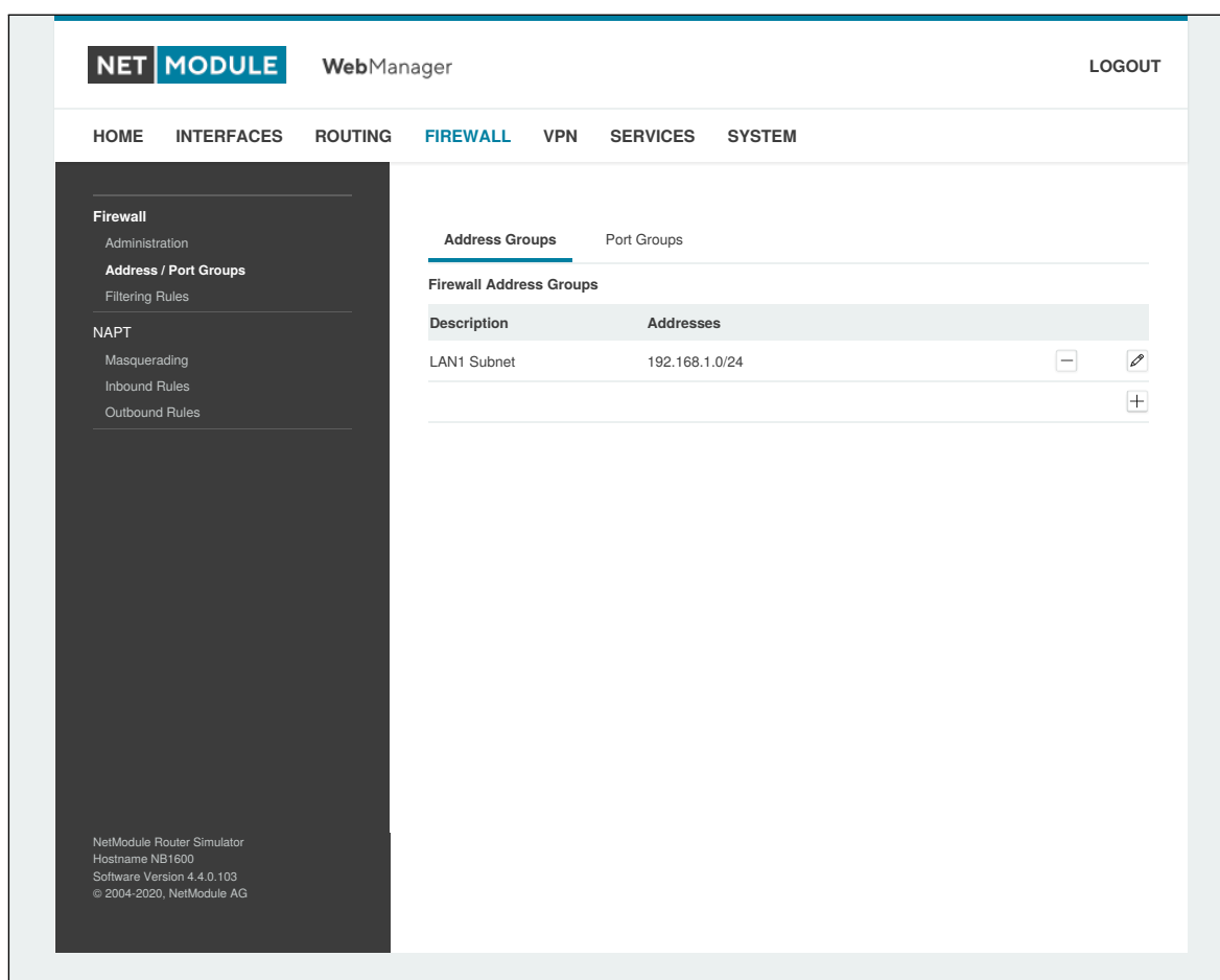
Abbildung 6.28.: Firewall-Gruppen
