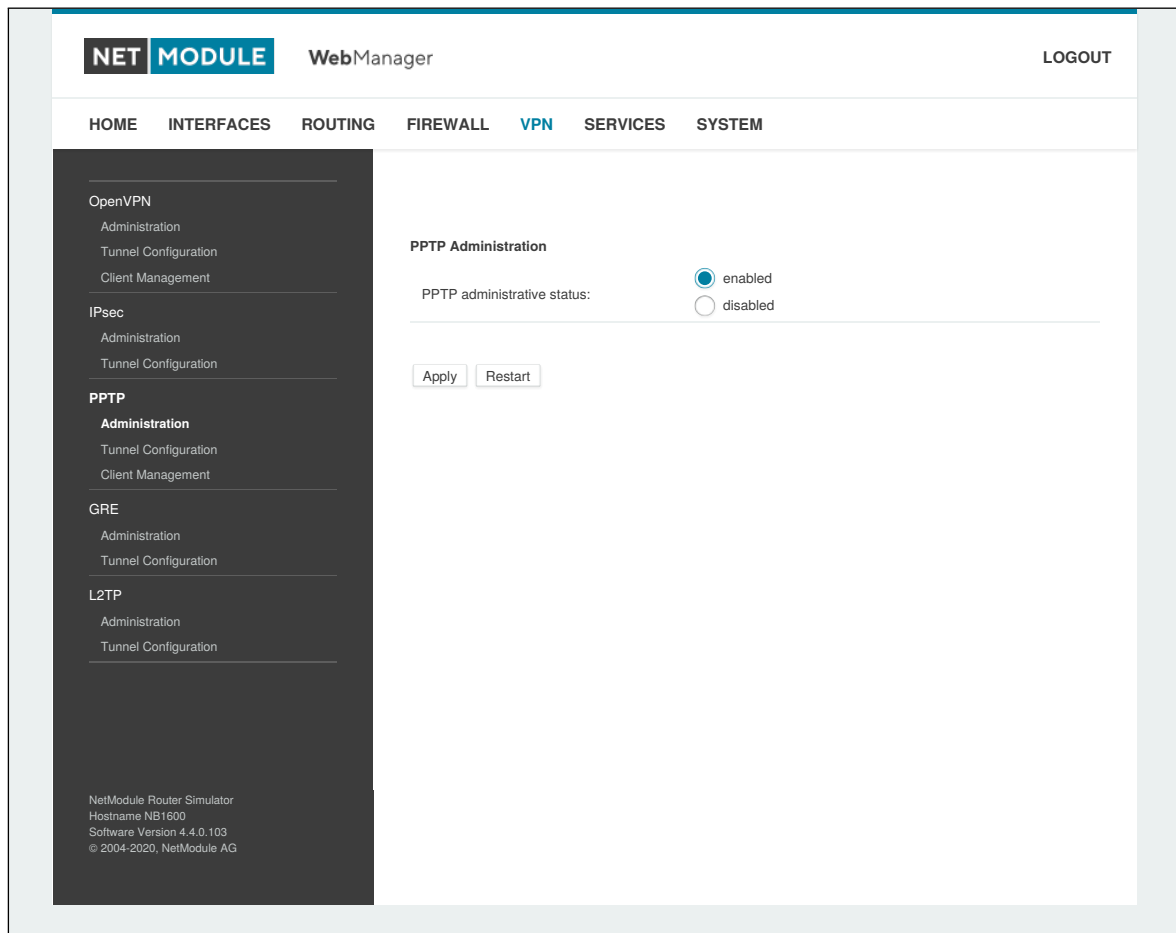
Abbildung 6.37.: PPTP-Verwaltung
