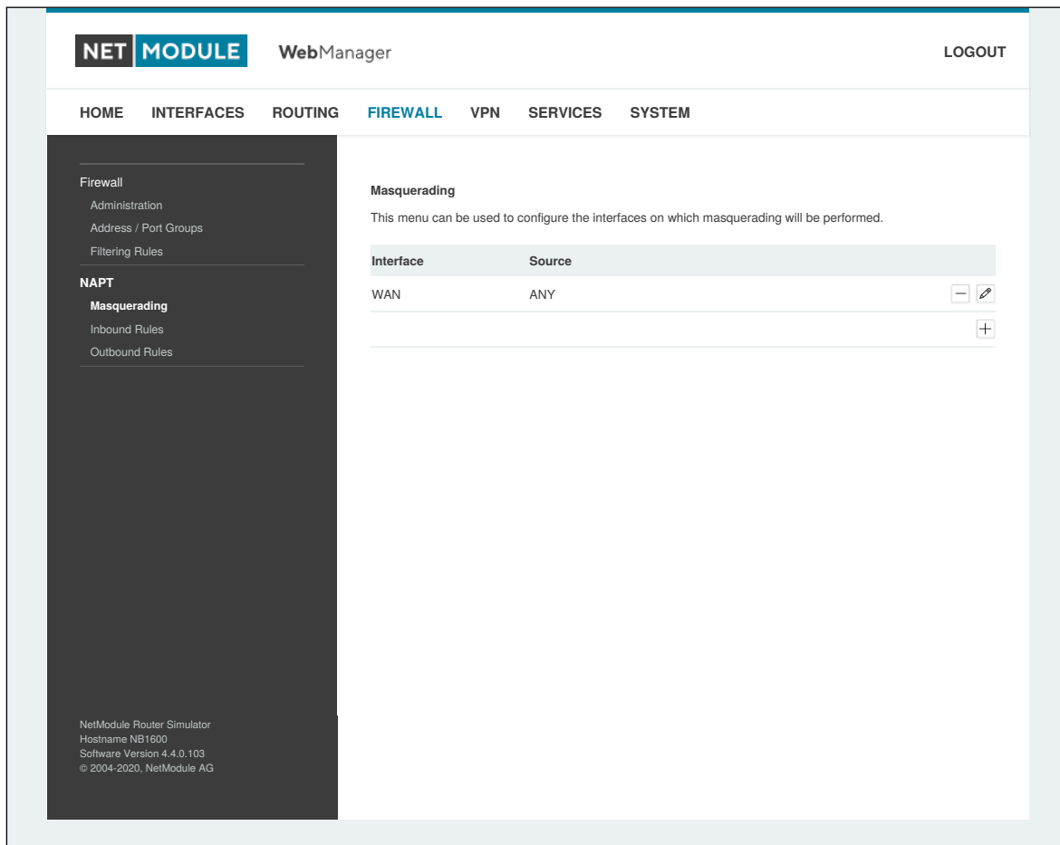
Abbildung 6.29.: Maskierung (Masquerading)
