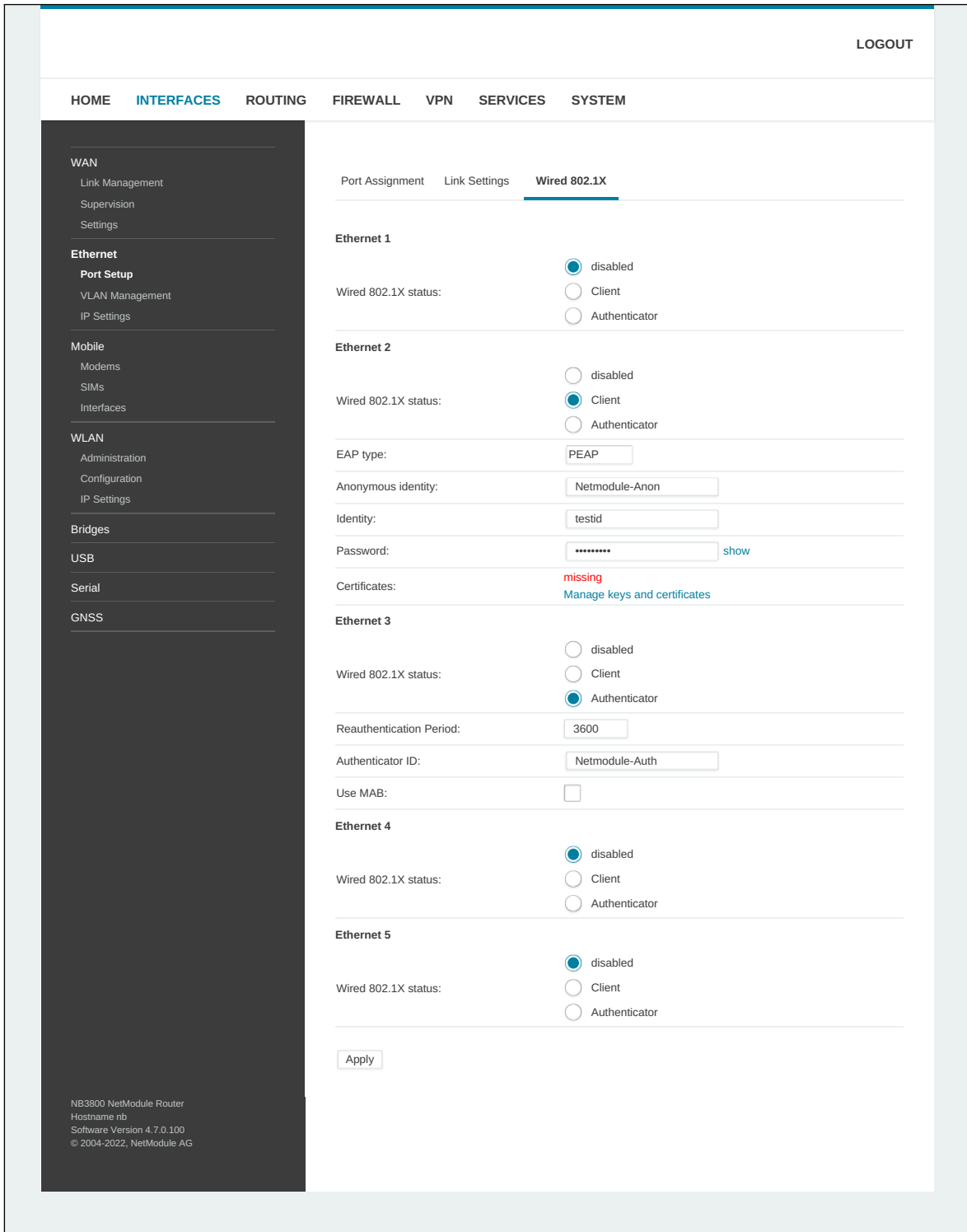
Abbildung 5.9.: Authentifizierung nach IEEE 802.1X
