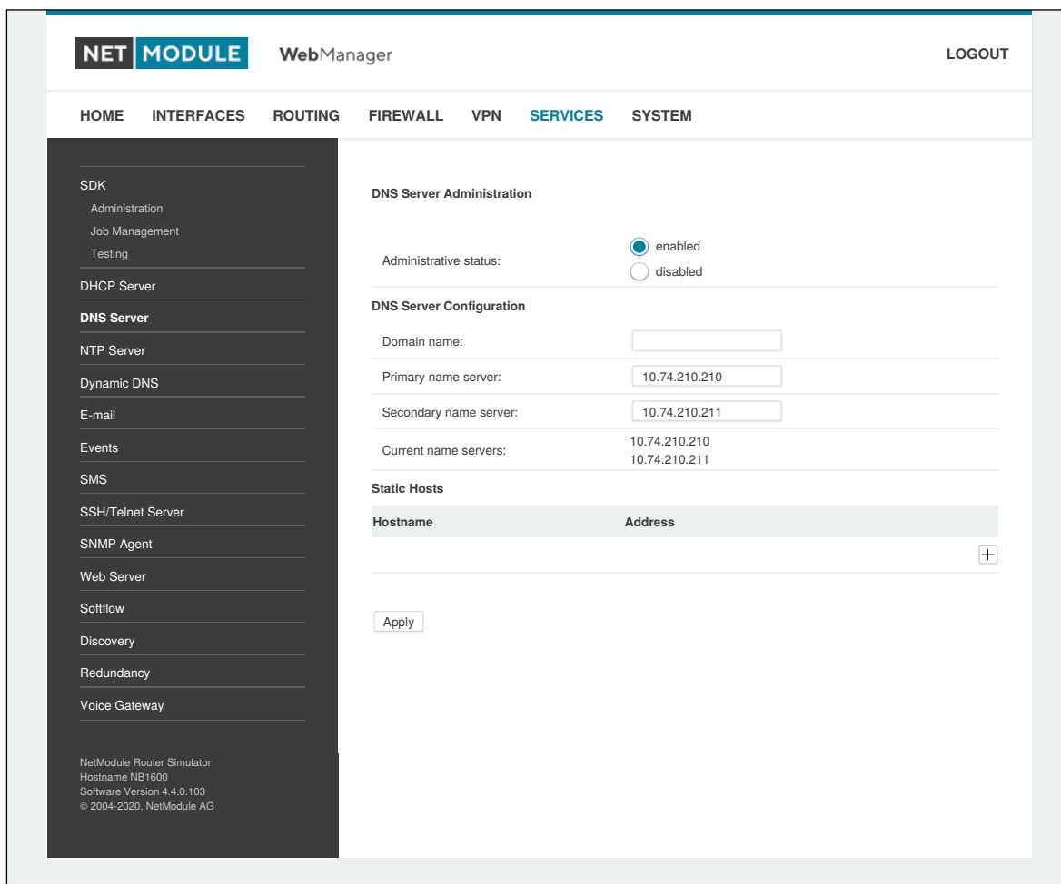
Abbildung 5.42.: DNS-Server
