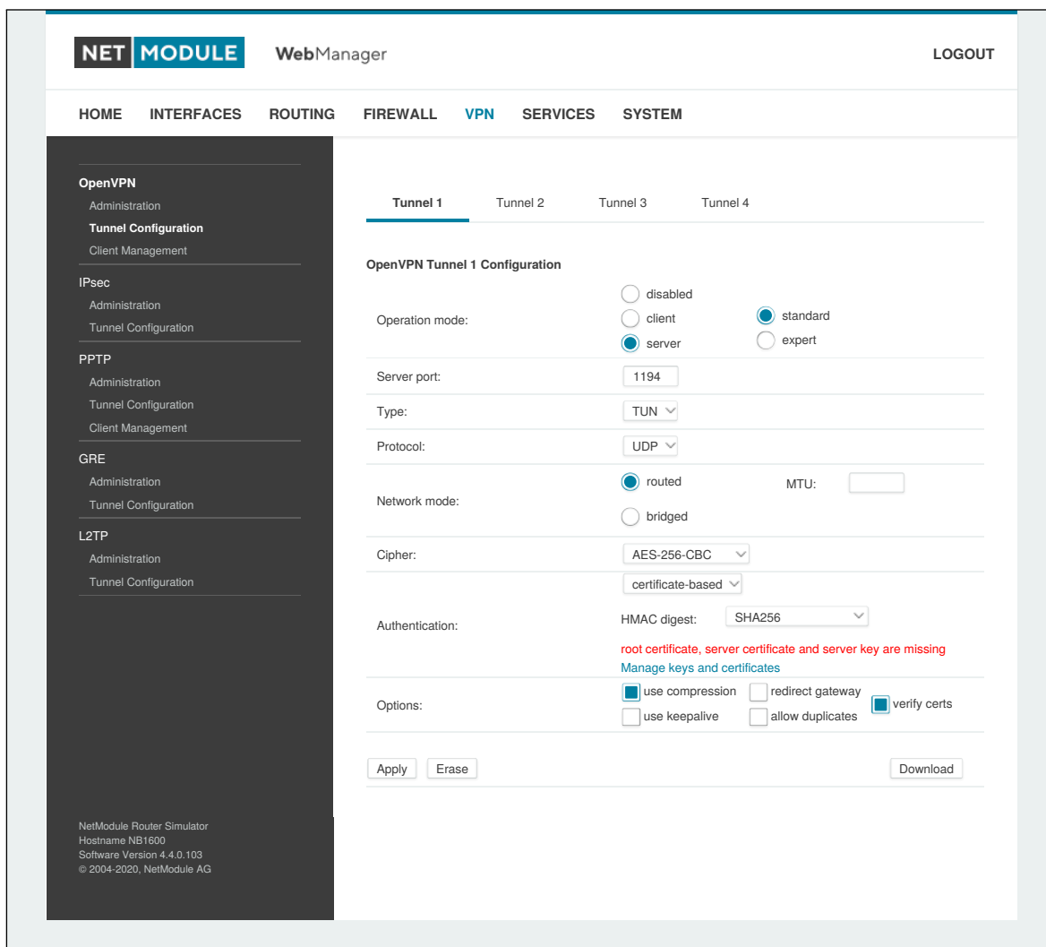
Abbildung 5.31.: Konfiguration von OpenVPN
