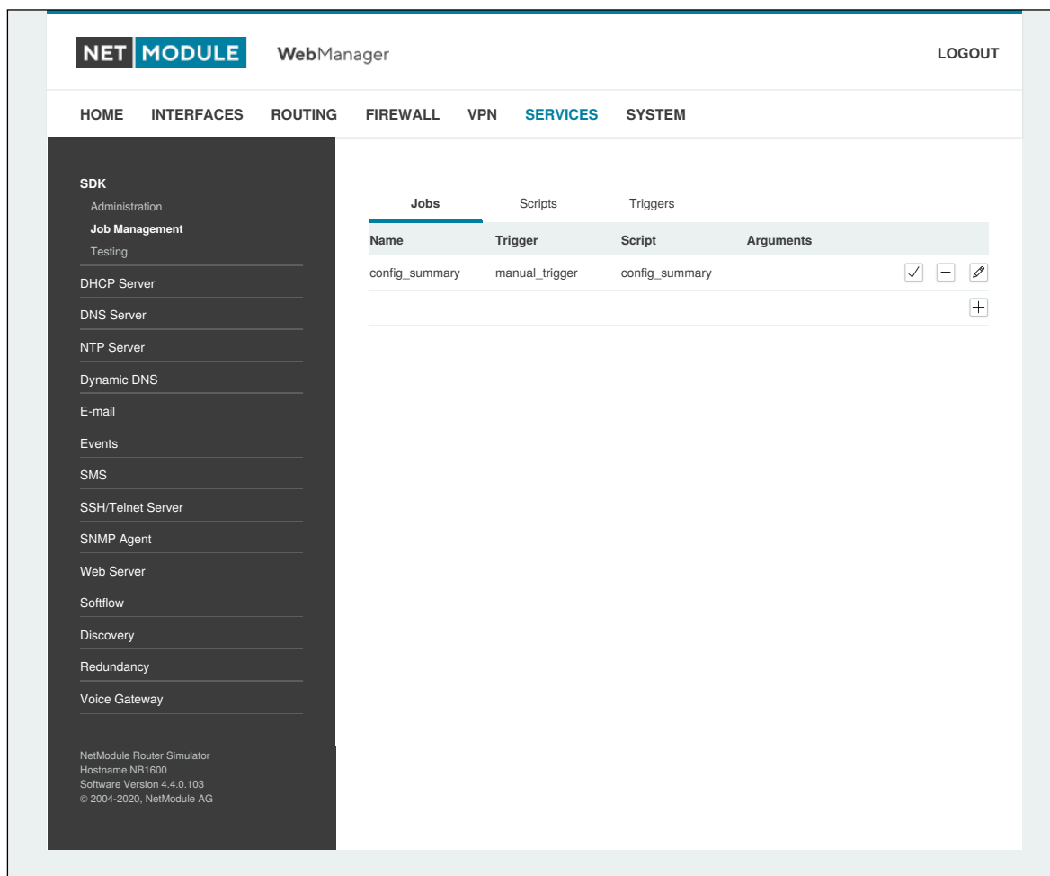
Abbildung 5.40.: SDK-Jobs
