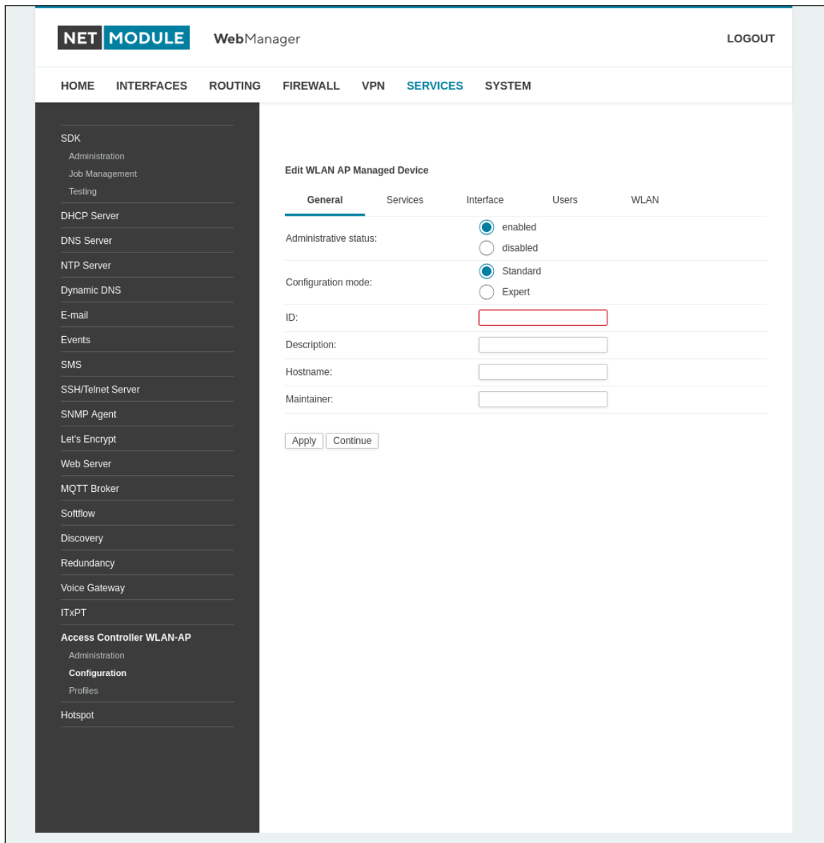
Abbildung 5.58.: AC WLAN-AP Configuration
