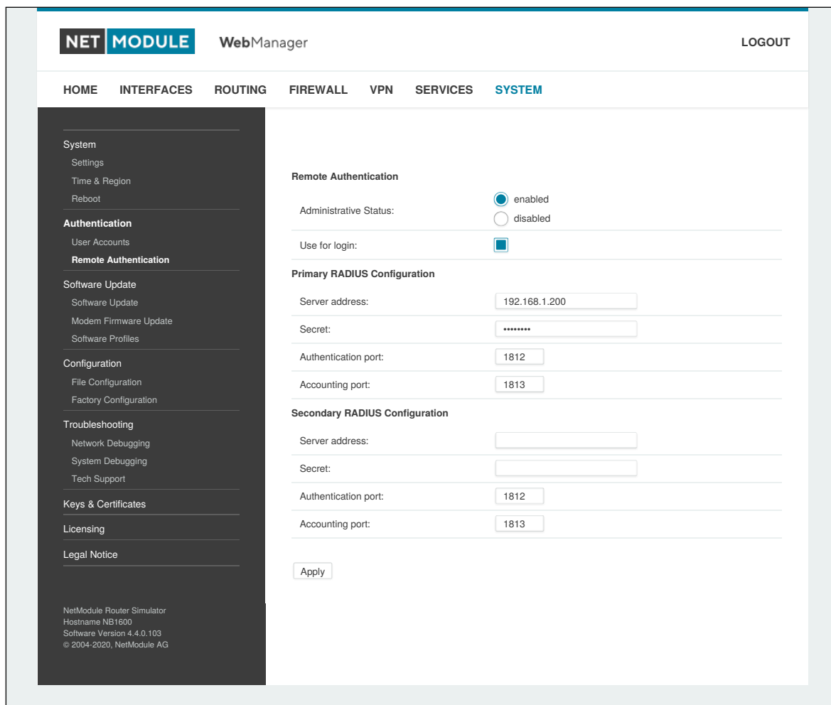
Abbildung 5.55.: Remote-Authentifizierung
