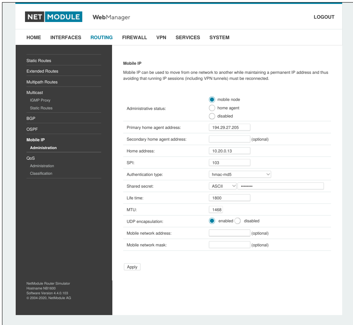
Abbildung 5.28.: Mobile IP
