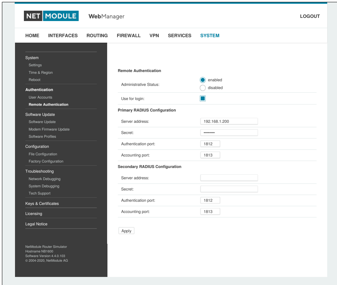
Abbildung 5.58.: Remote-Authentifizierung
