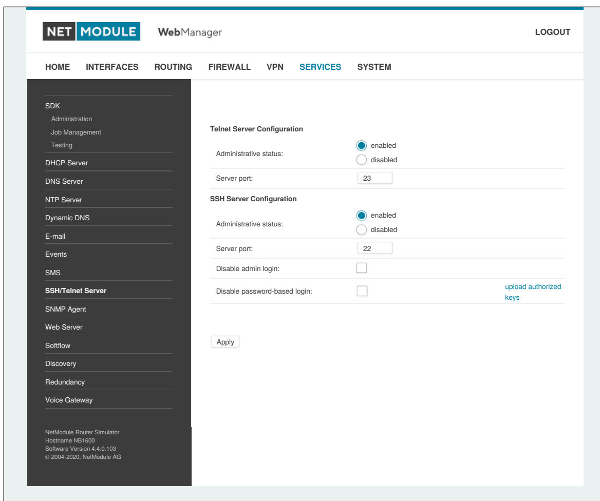
Abbildung 5.50.: SSH- und Telnet-Server
