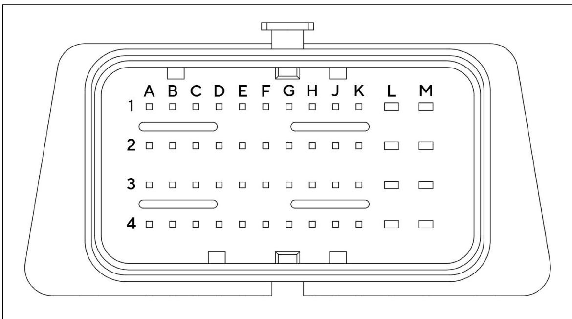
Abbildung 3.4.: X48 Outline
