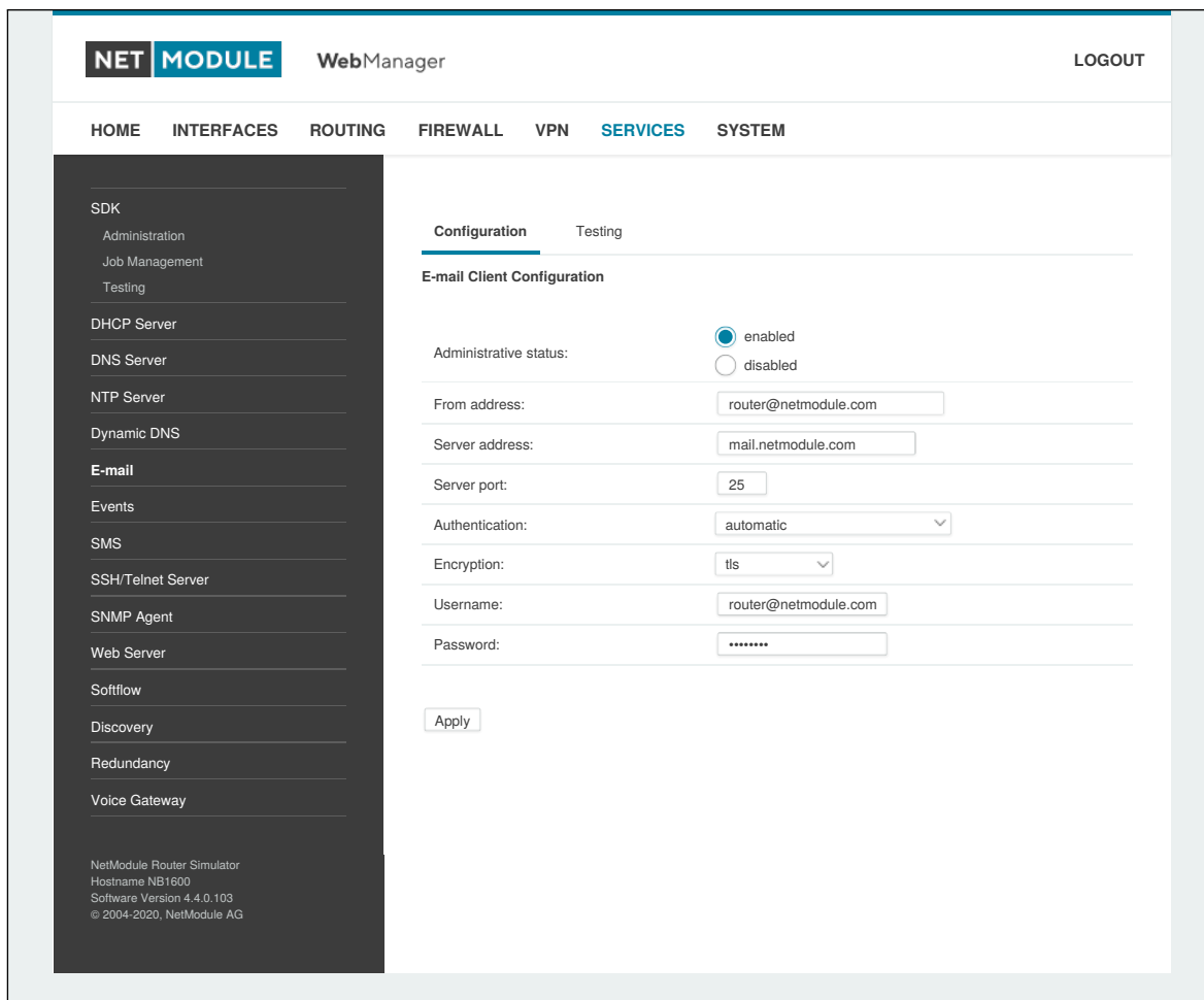
Abbildung 5.45.: E-Mail-Einstellungen
