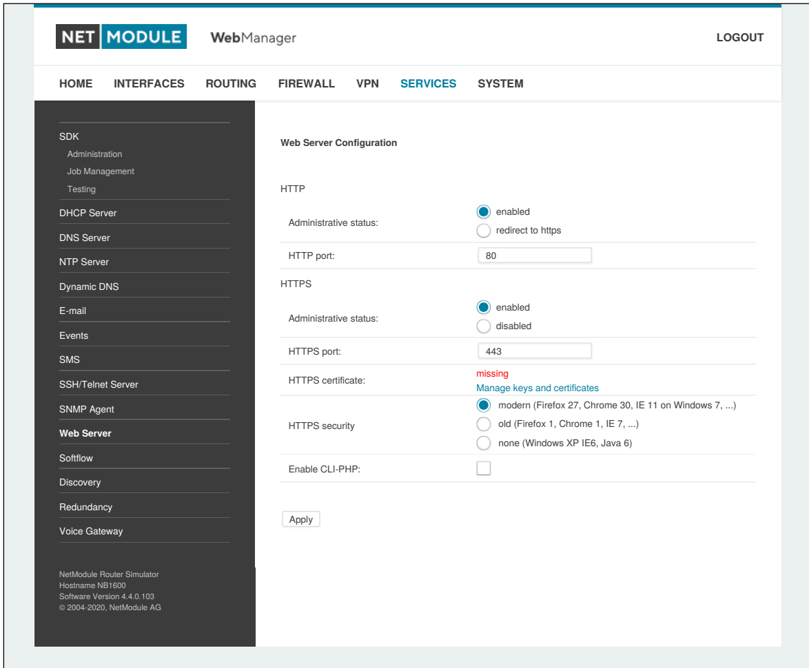
Abbildung 5.49.: Webserver
