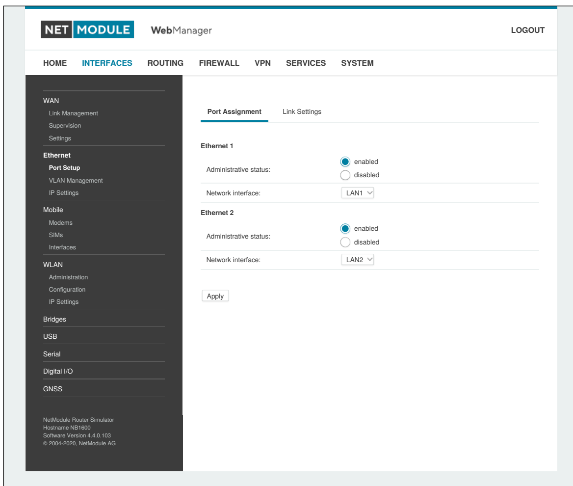
Abbildung 5.6.: Ethernet-Anschlüsse
