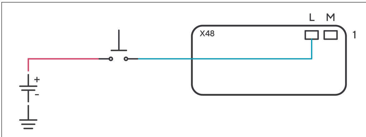
Abbildung 3.1.: Reset-Eingang (serielle Schnittstelle nicht verwendet)
