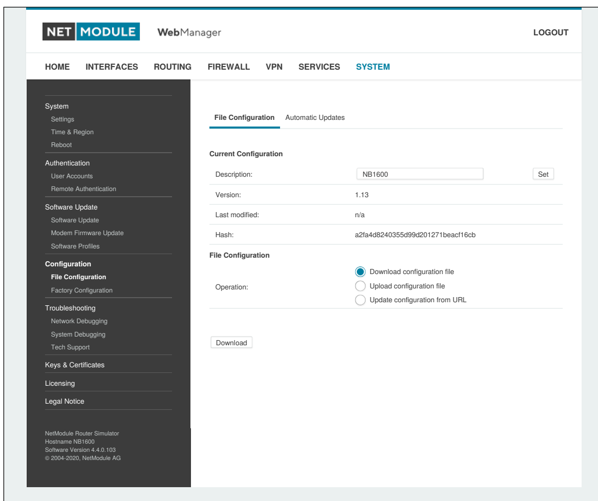
Abbildung 5.60.: Manuelle Konfiguration per Datei
