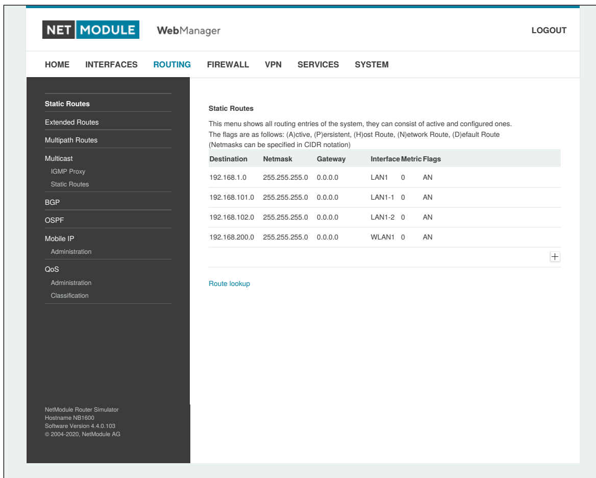
Abbildung 5.21.: Statisches Routing
