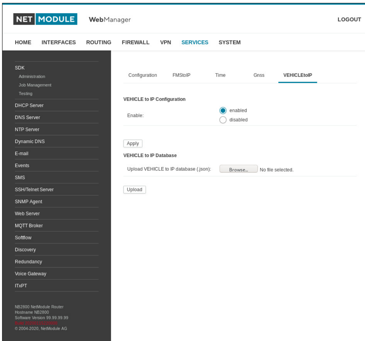
Abbildung 5.54.: ITxPT VEHICLEtoIP
