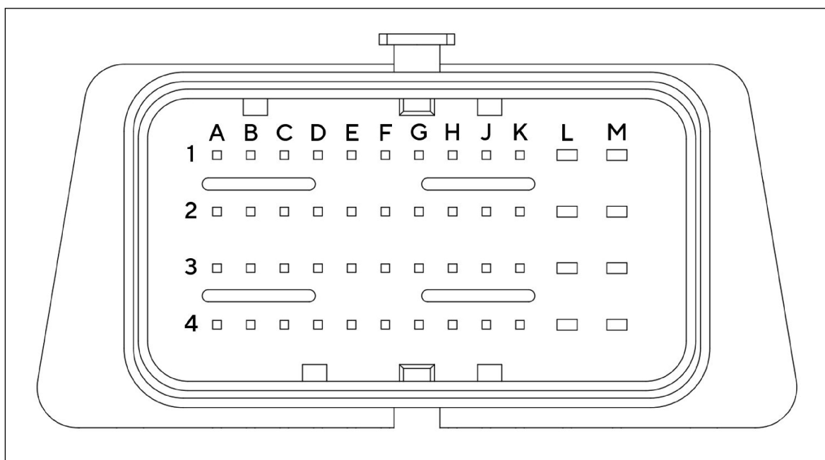
Abbildung 3.4.: X48 Outline
