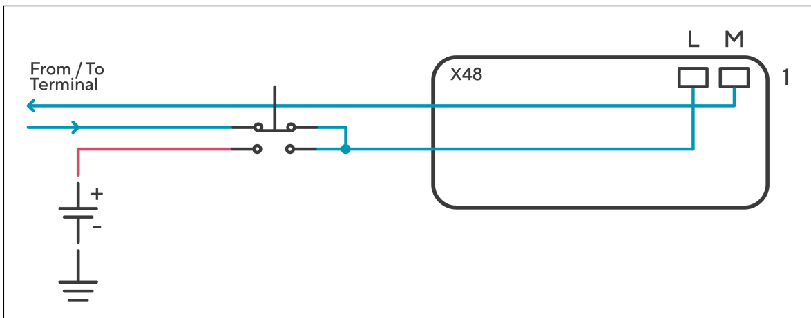
Abbildung 3.2.: Reset-Eingang (serielle Schnittstelle verwendet)
