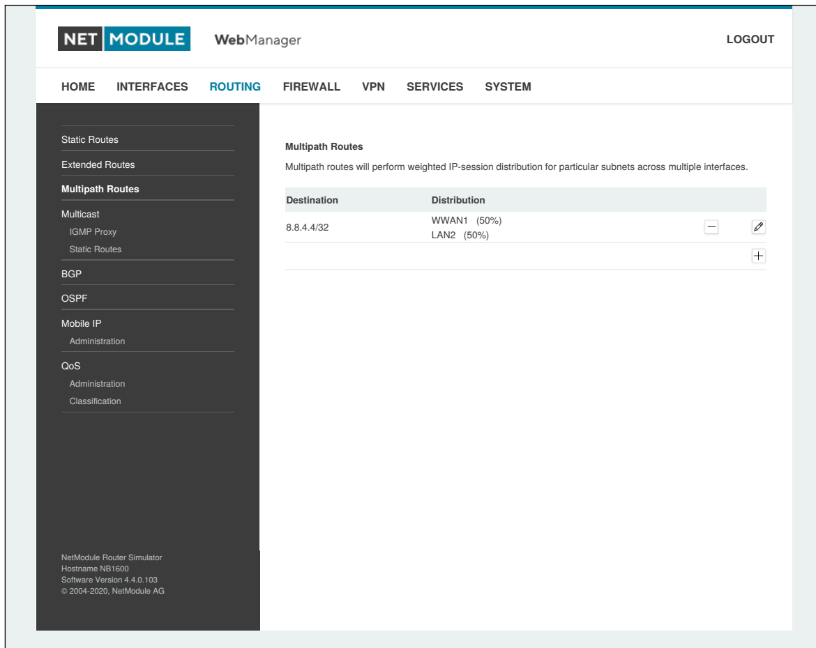
Abbildung 5.25.: Multipath-Routing
