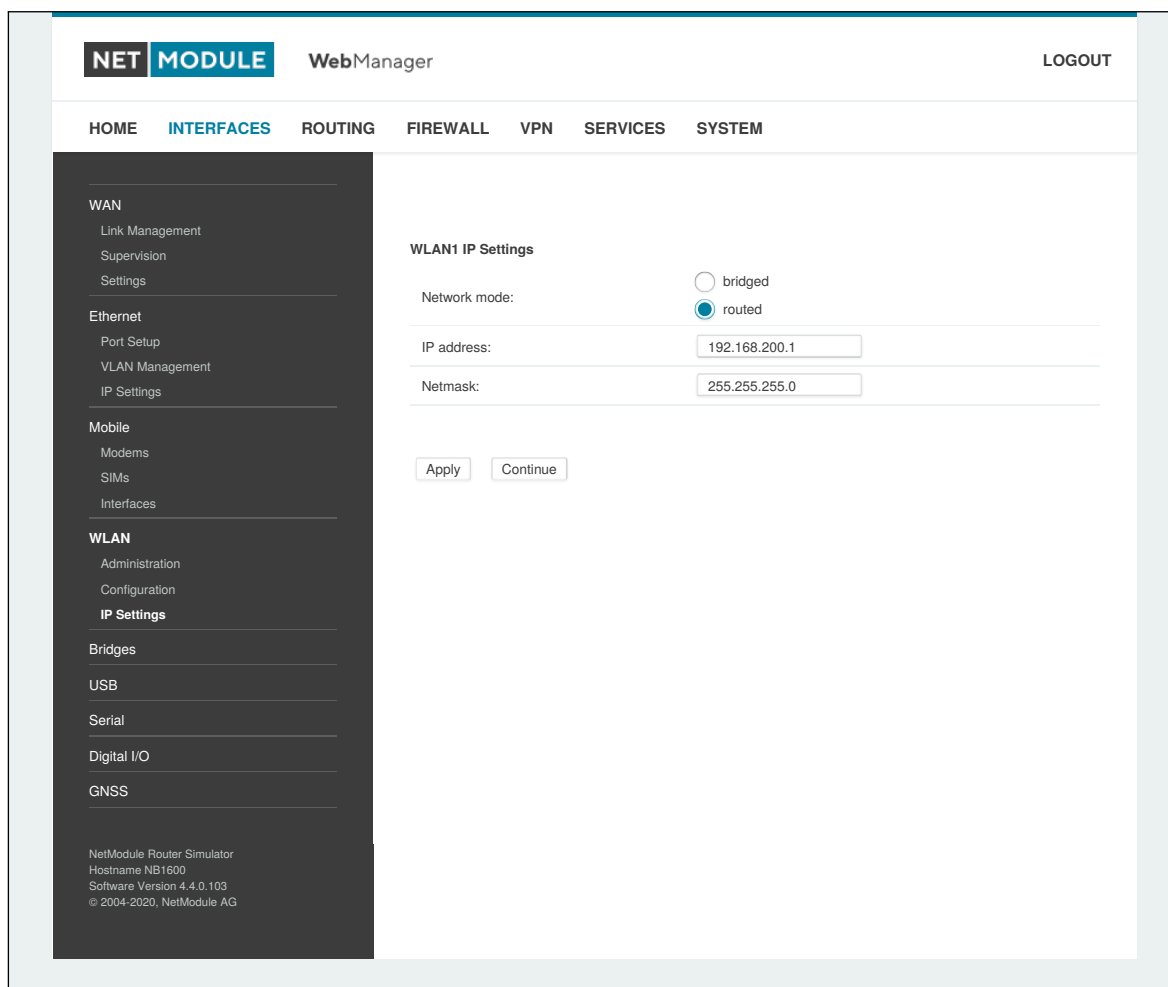
Abbildung 5.21.: WLAN-IP-Konfiguration
