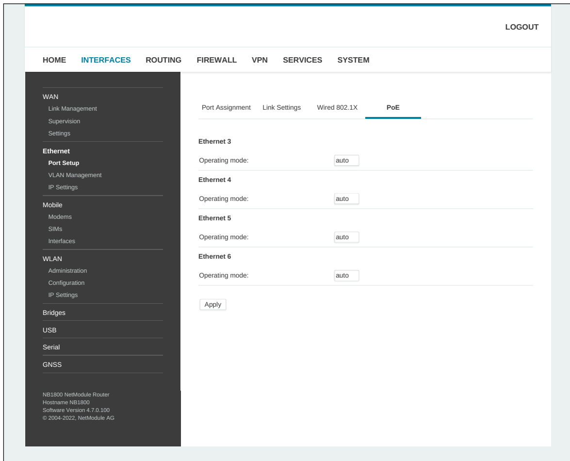
Abbildung 5.10.: PoE-Power-Supply
