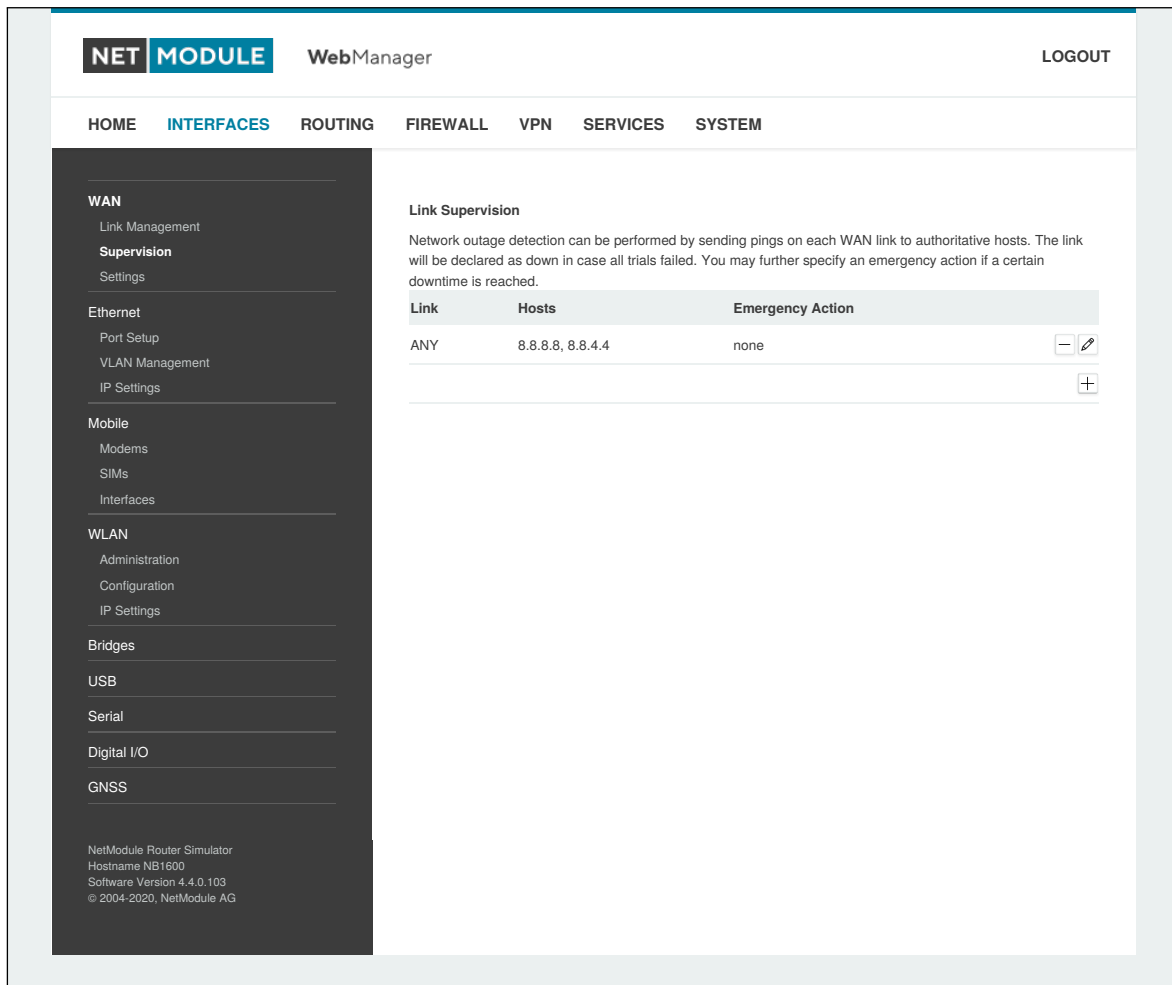
Abbildung 6.5.: Verbindungsüberwachung
