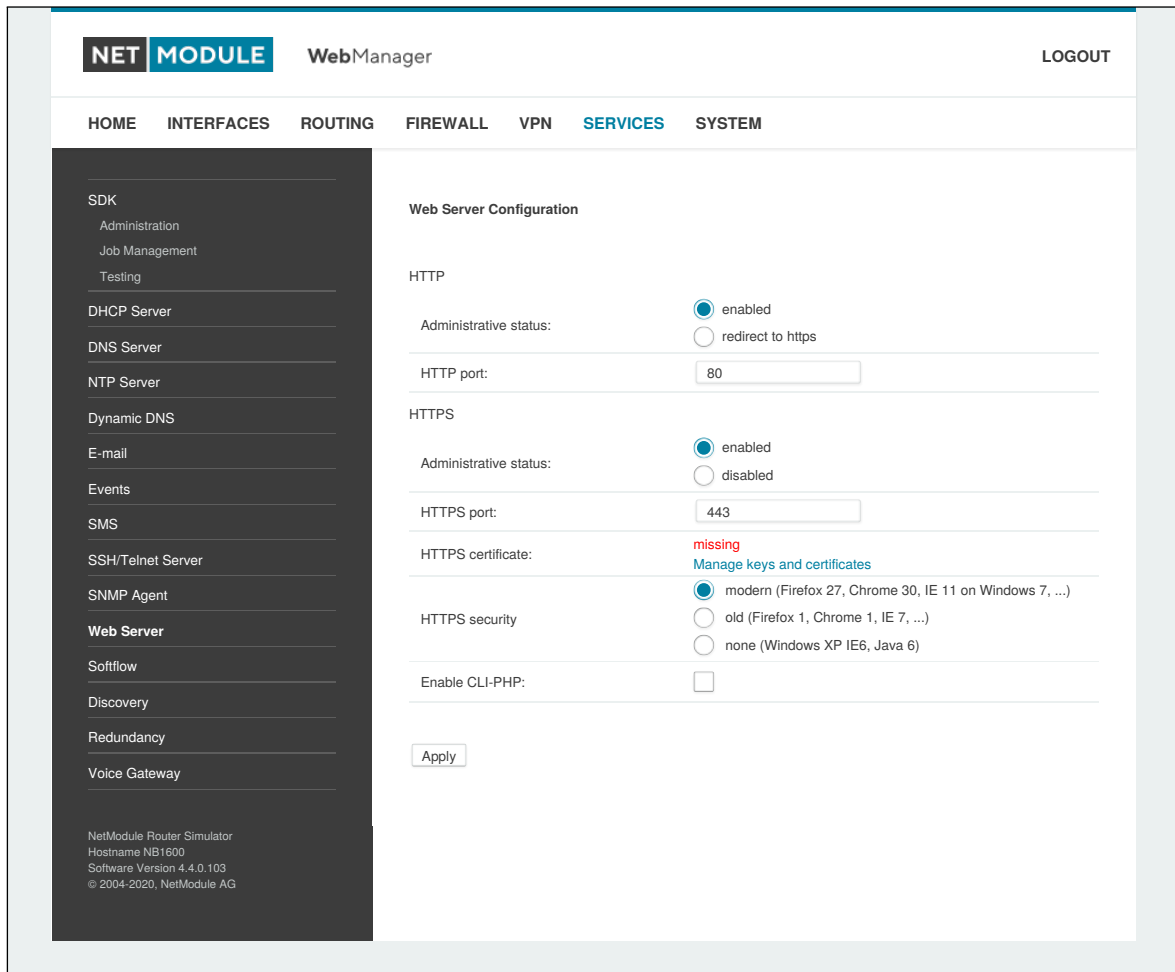
Abbildung 6.51.: Webserver
