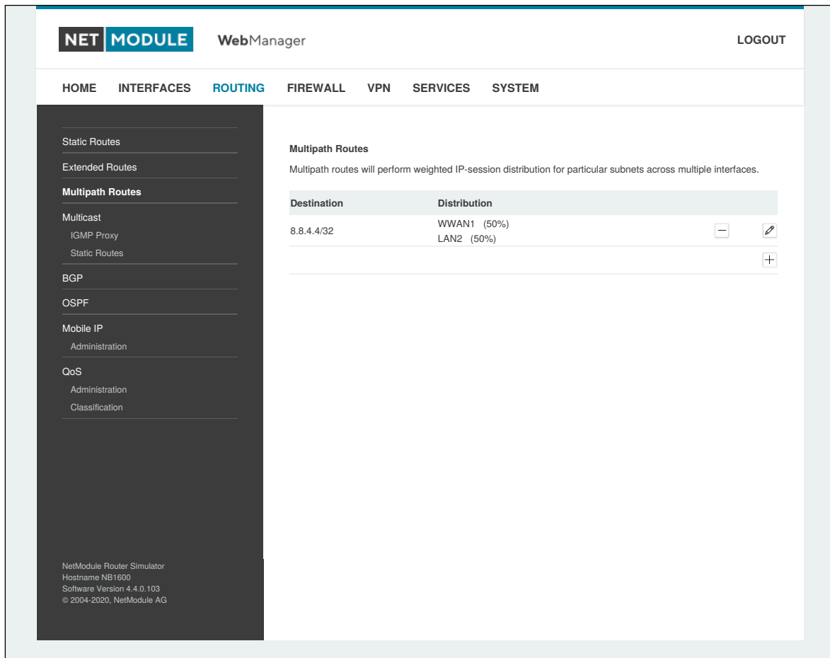
Abbildung 6.27.: Multipath-Routing
