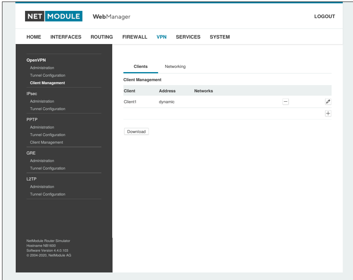
Abbildung 6.32.: OpenVPN-Client-Verwaltung
