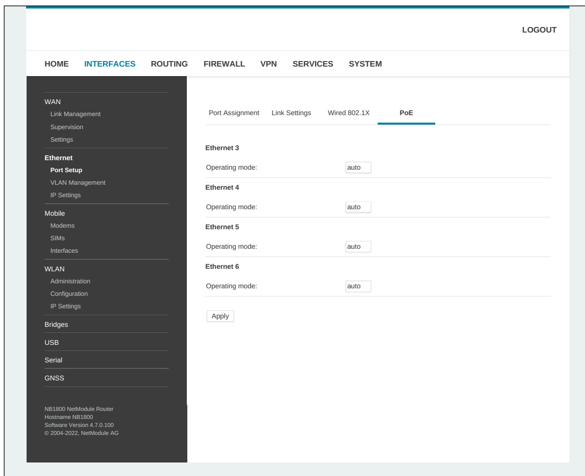
Abbildung 6.10.: PoE-Power-Supply
