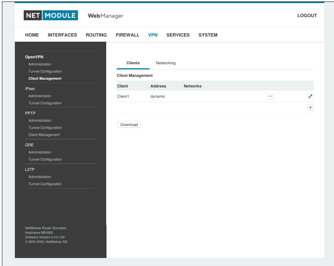
Abbildung 6.36.: OpenVPN-Client-Verwaltung
