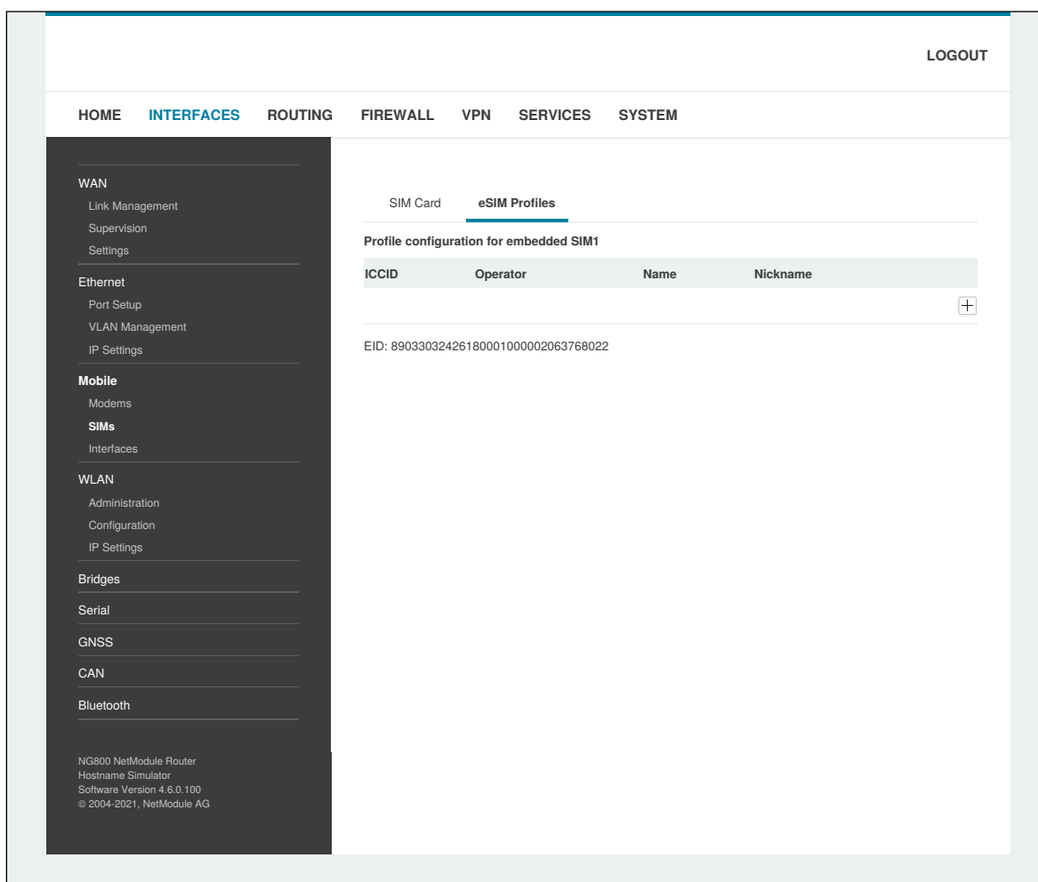
Abbildung 6.16.: eSIM-Profilen
