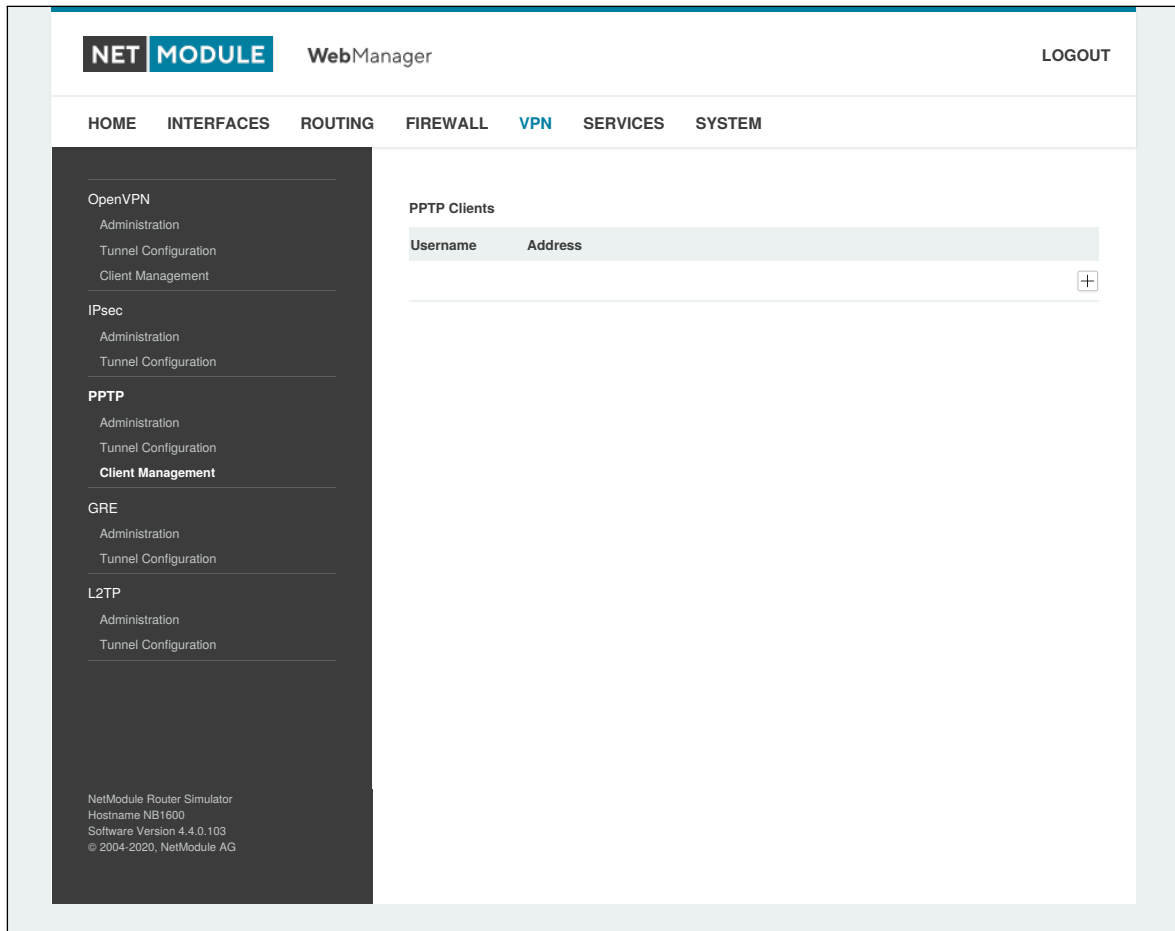
Abbildung 6.41.: PPTP-Client-Verwaltung
