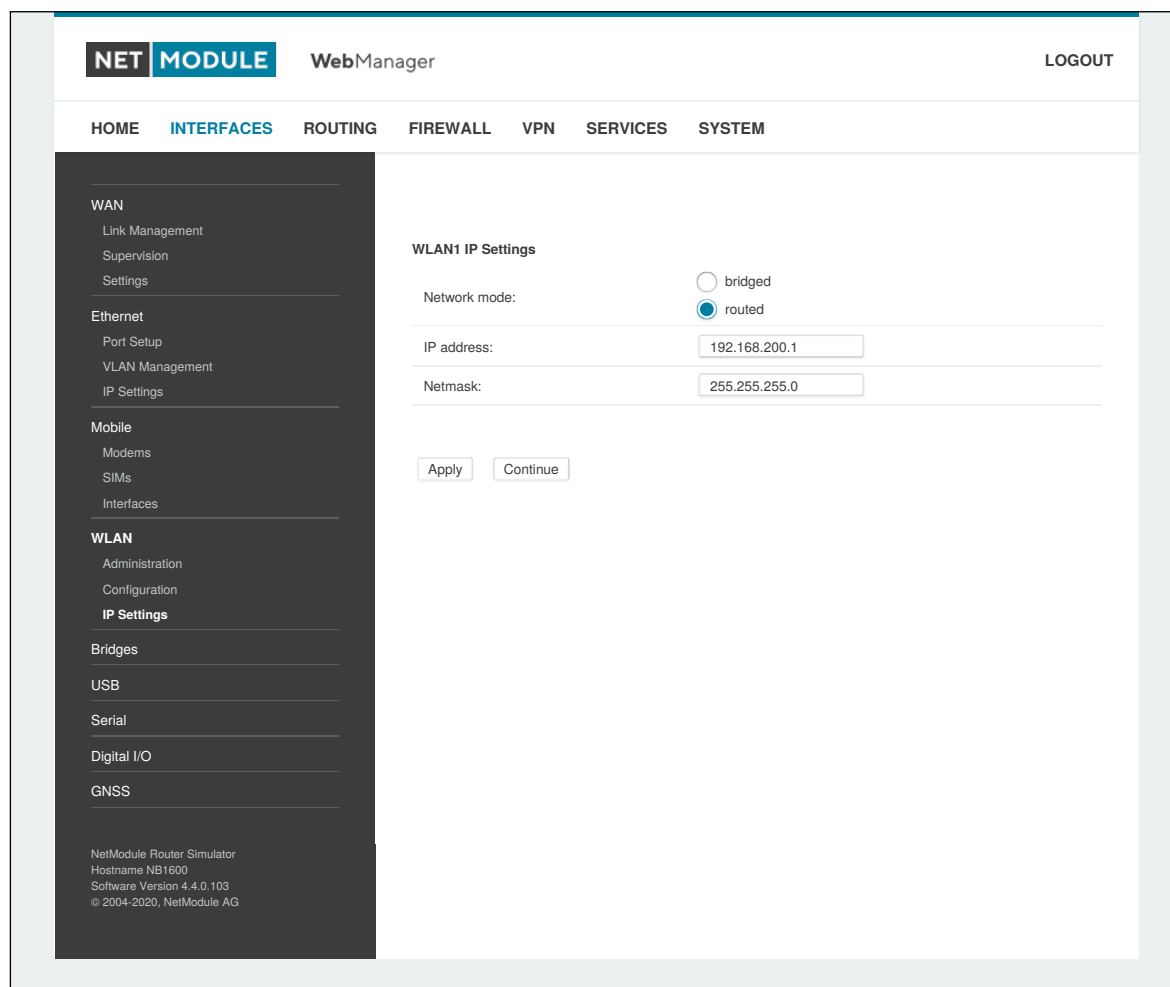
Abbildung 6.21.: WLAN-IP-Konfiguration
