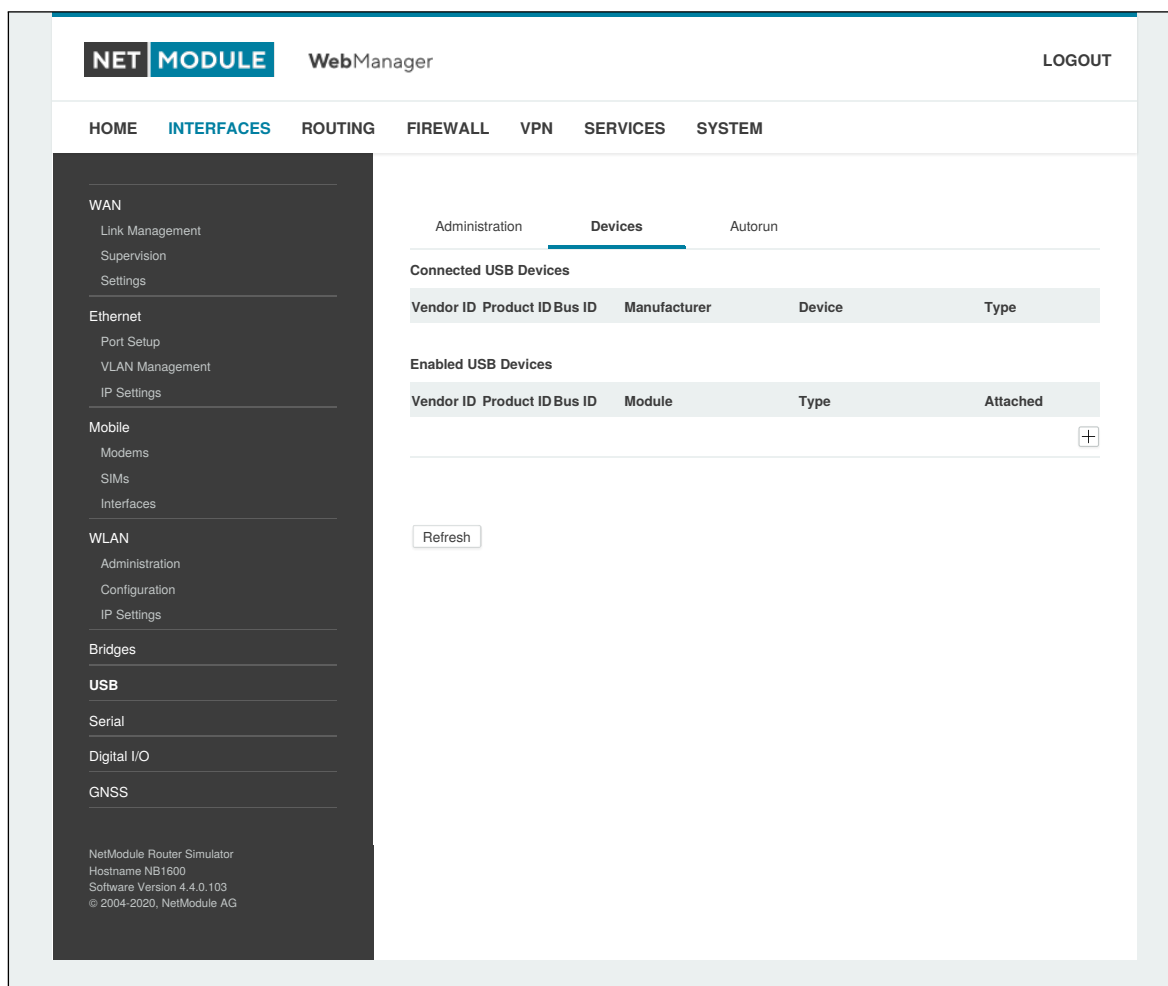
Abbildung 6.23.: USB-Geräteverwaltung
