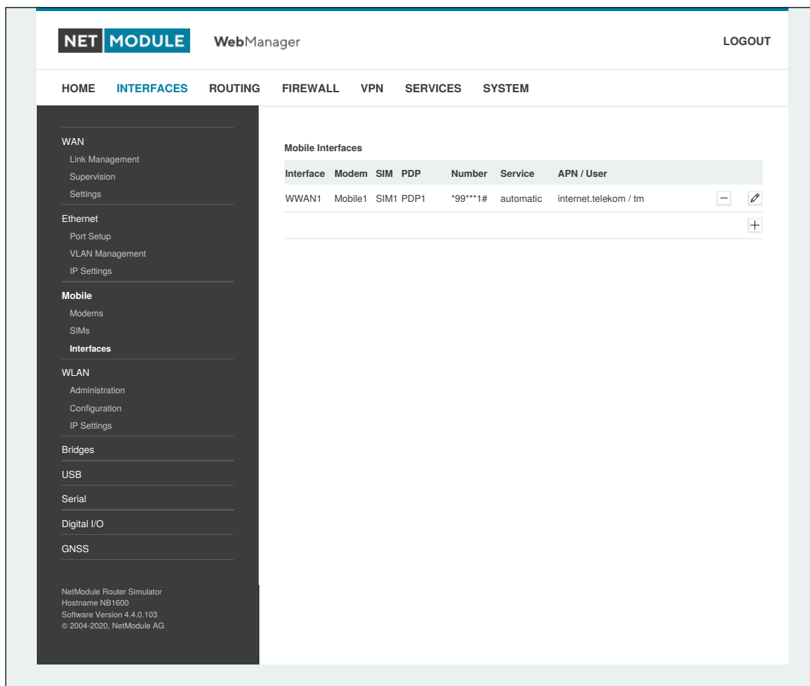
Abbildung 6.16.: WWAN-Schnittstellen
