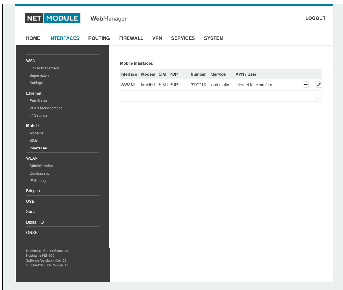
Abbildung 6.16.: WWAN-Schnittstellen
