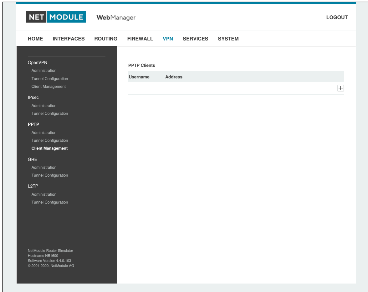
Abbildung 6.37.: PPTP-Client-Verwaltung
