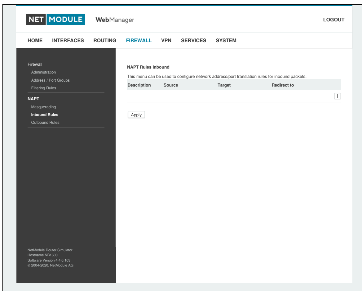
Abbildung 6.29.: NAPT-Regeln für eingehende Pakete
