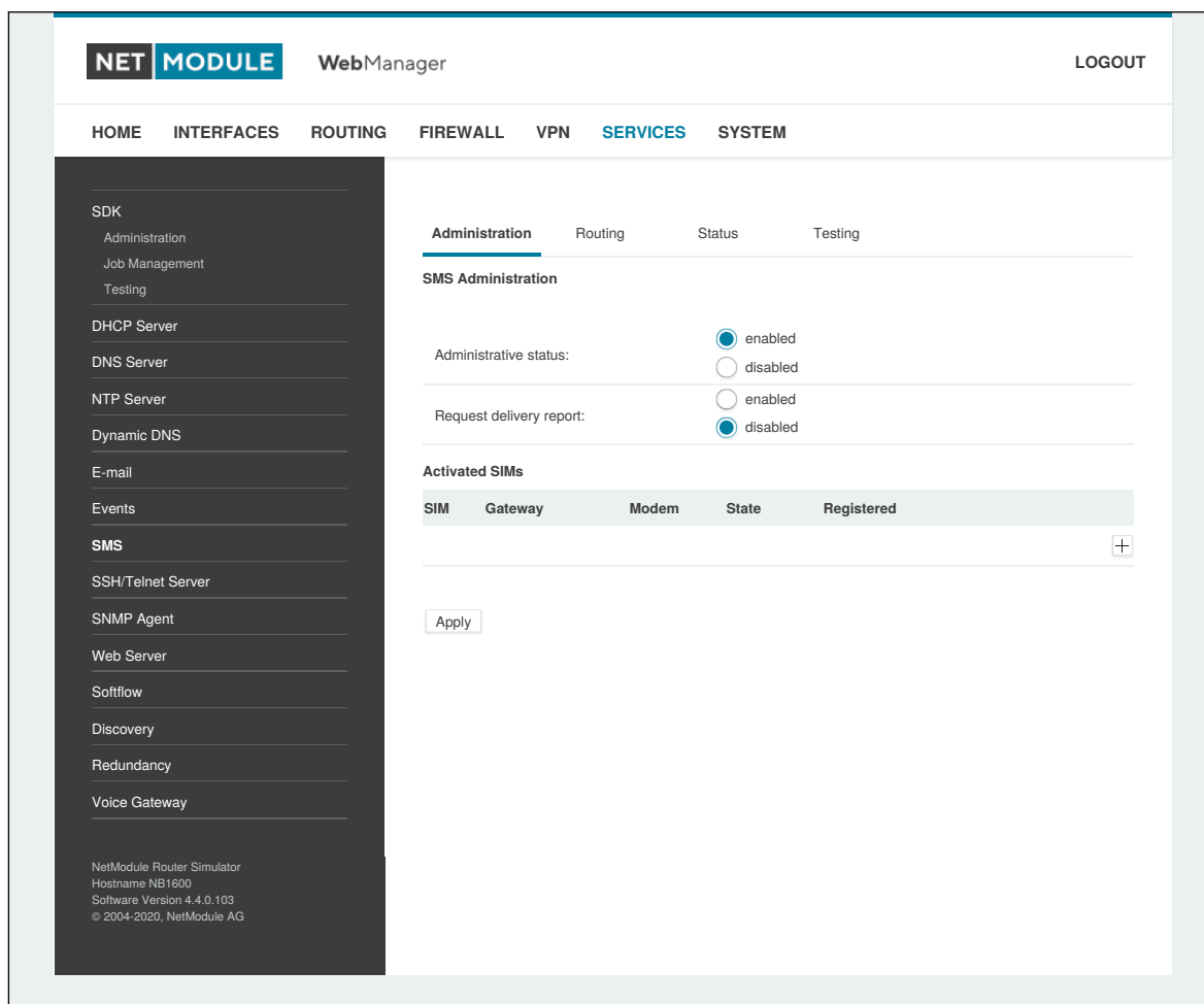
Abbildung 6.46.: SMS-Konfiguration
