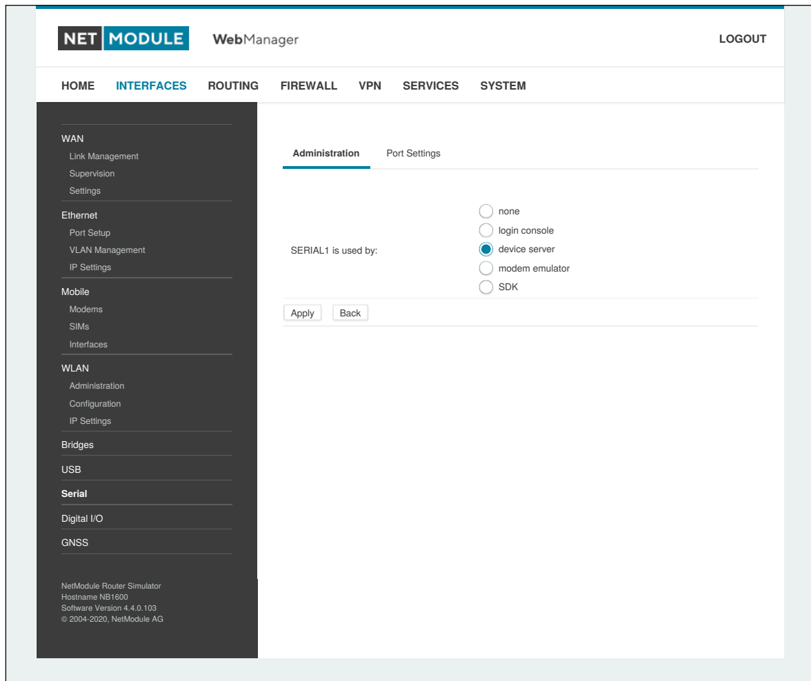
Abbildung 6.20.: Verwaltung der seriellen Schnittstelle
