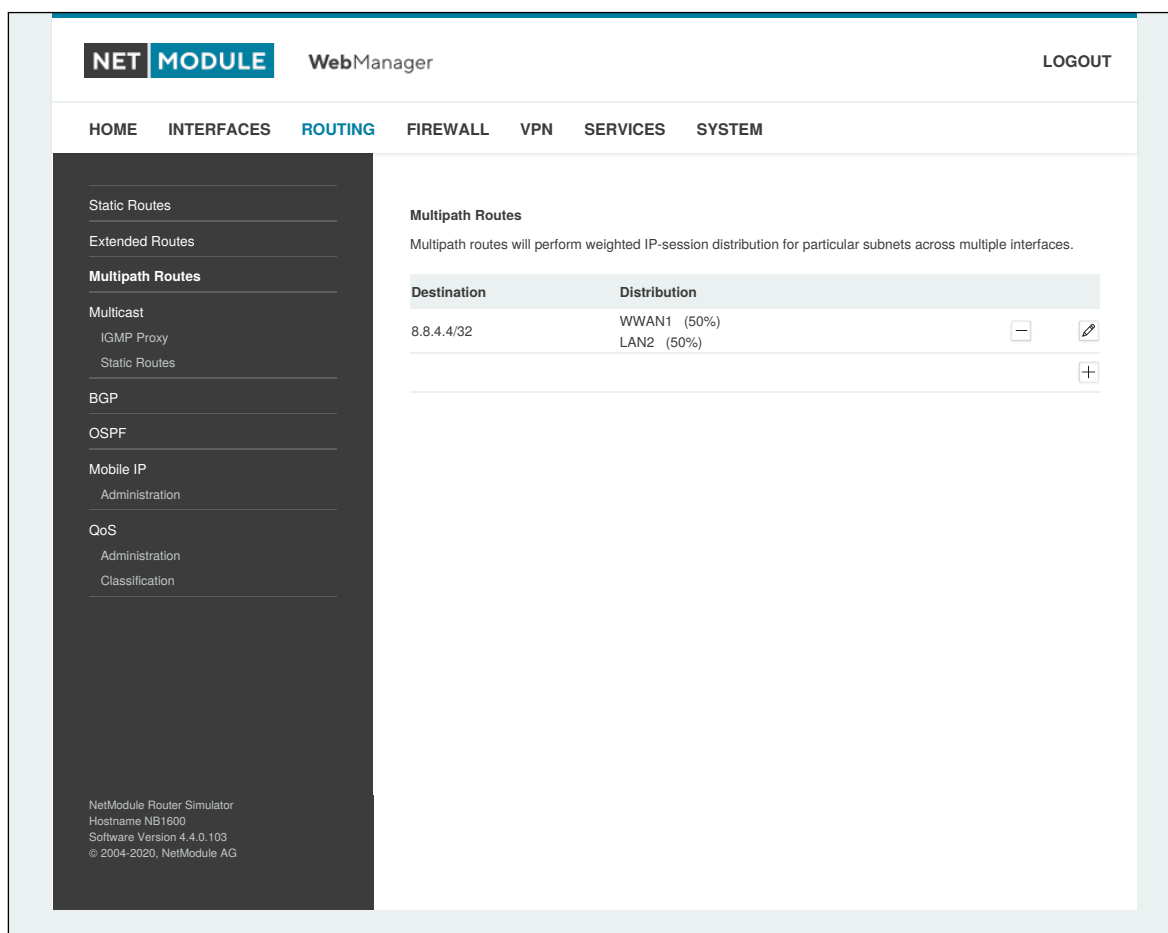
Abbildung 6.24.: Multipath-Routing
