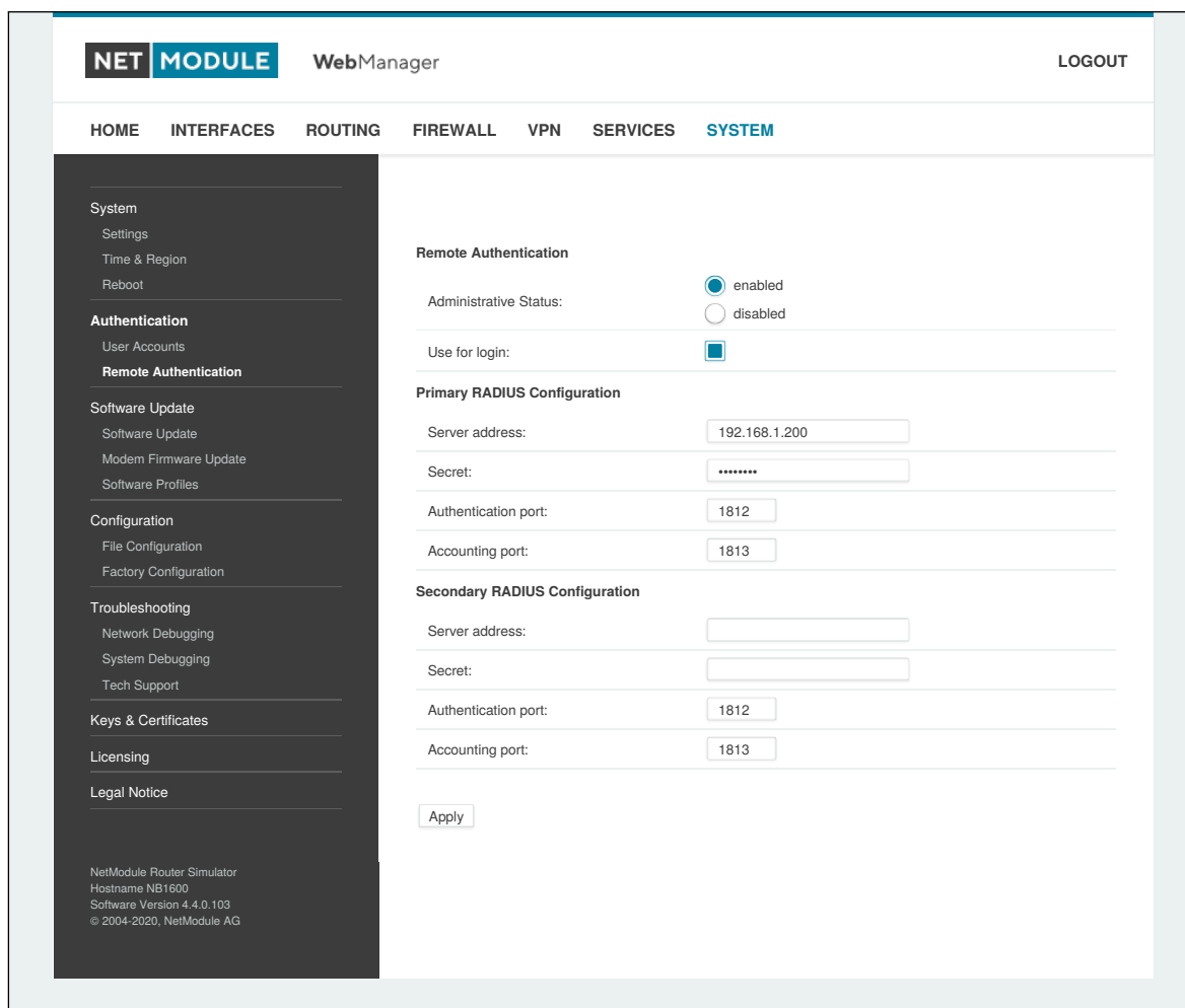
Abbildung 6.66.: Remote-Authentifizierung
