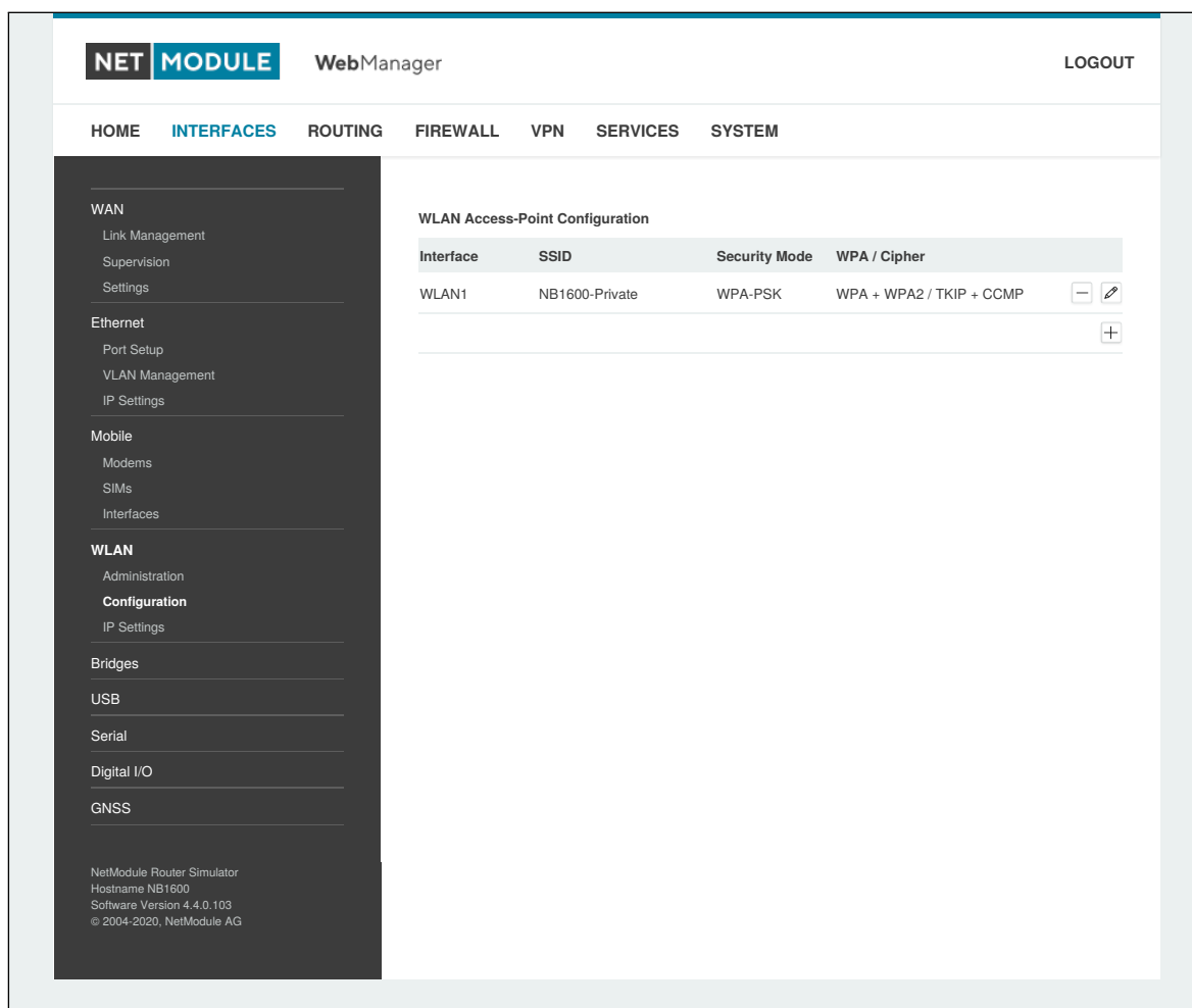
Abbildung 6.18.: WLAN-Konfiguration
