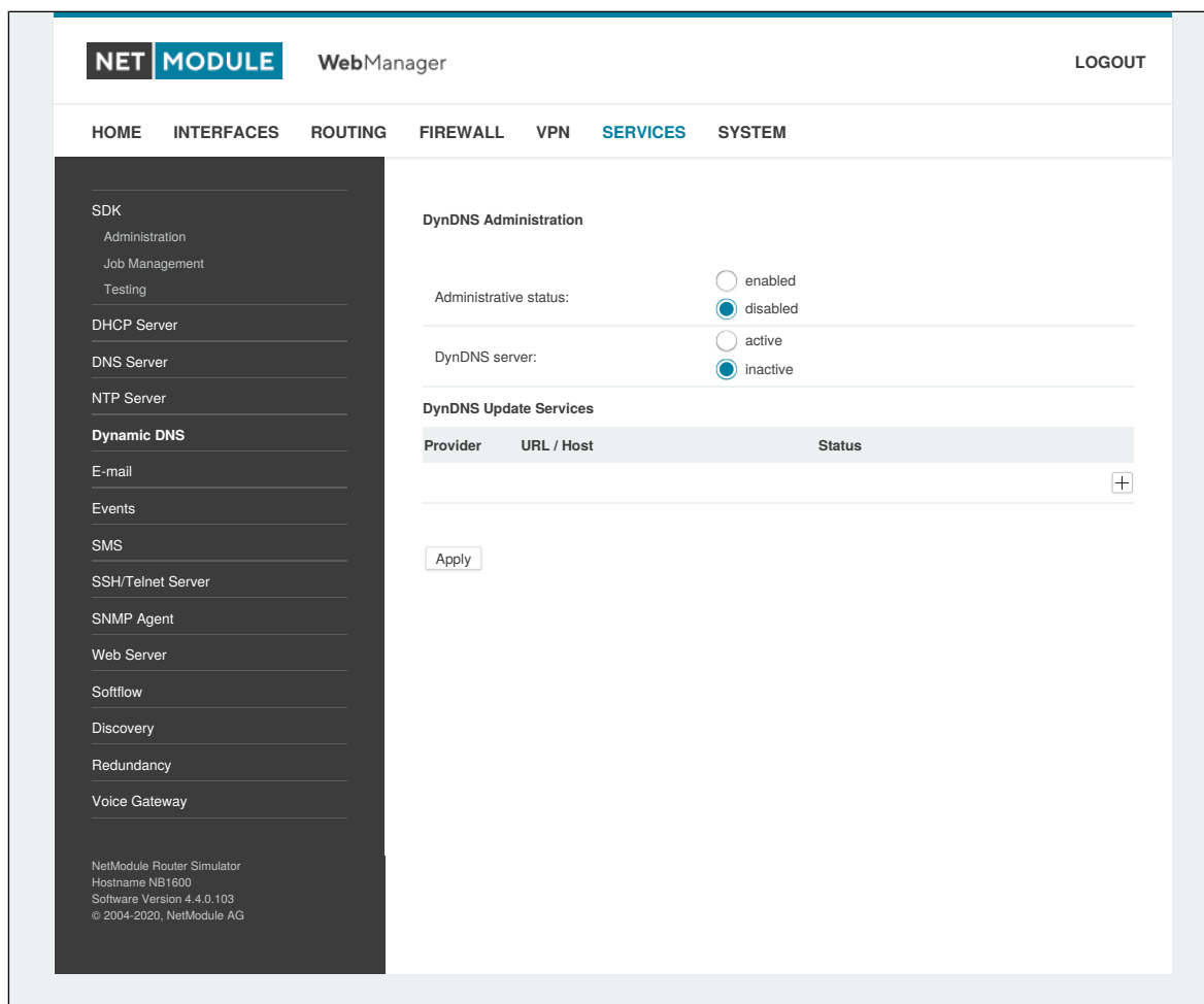
Abbildung 6.44.: Einstellungen für Dynamic DNS
