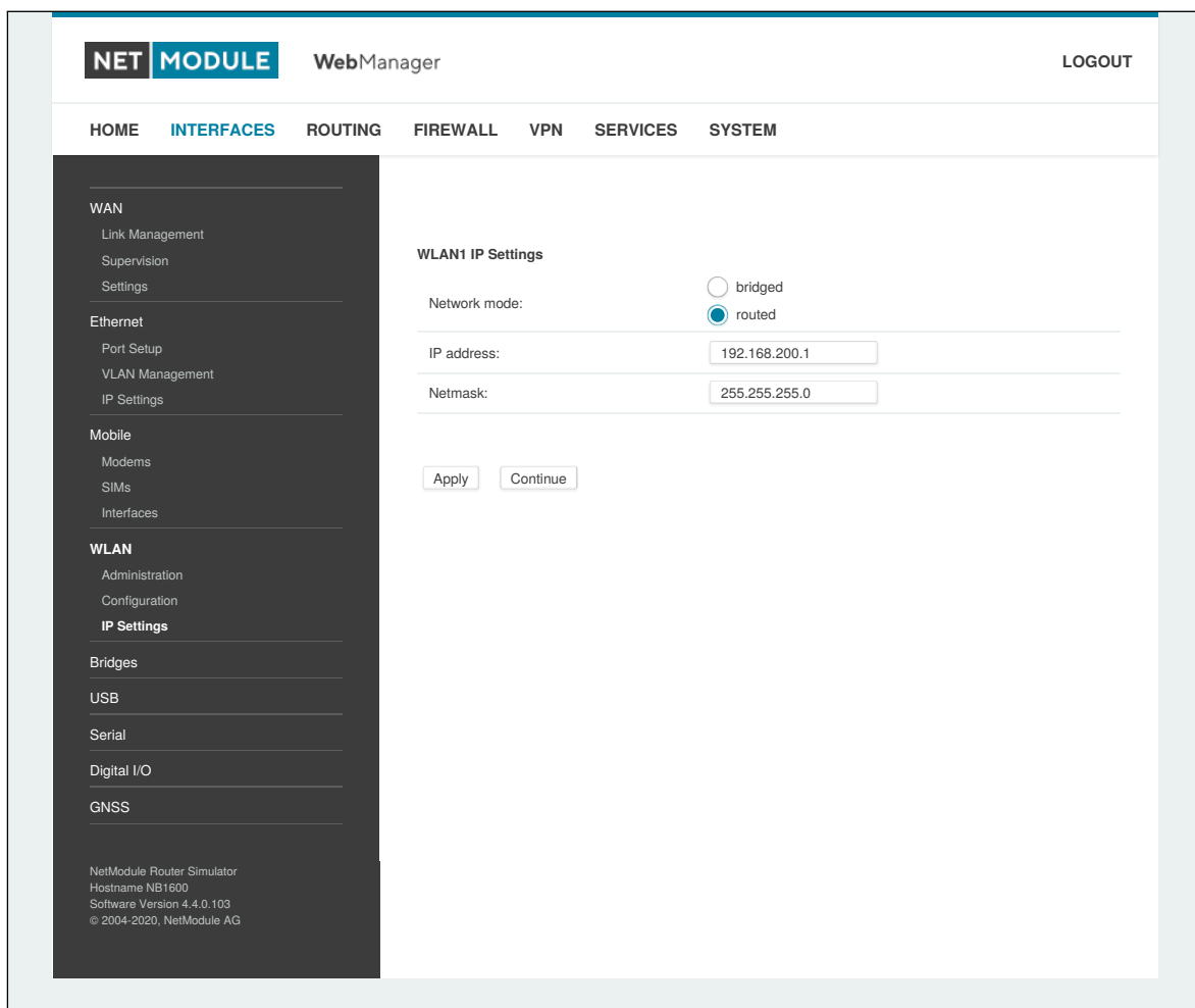
Abbildung 6.18.: WLAN-IP-Konfiguration
