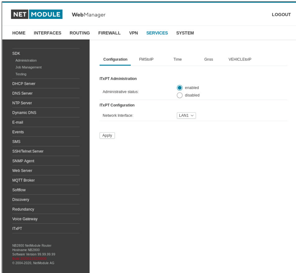
Abbildung 6.52.: ITxPT-Konfiguration
