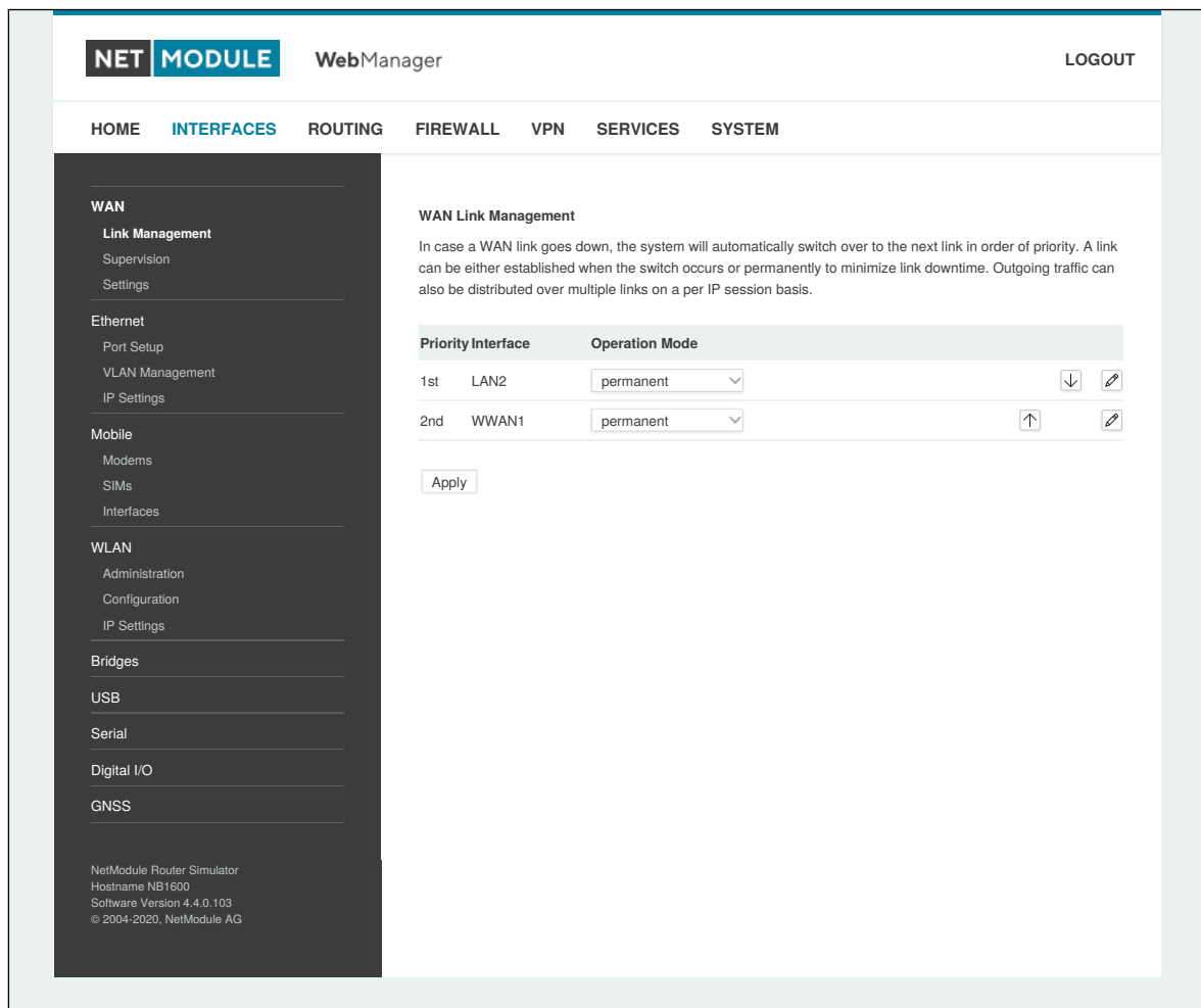
Abbildung 6.2.: WAN-Verbindungen
