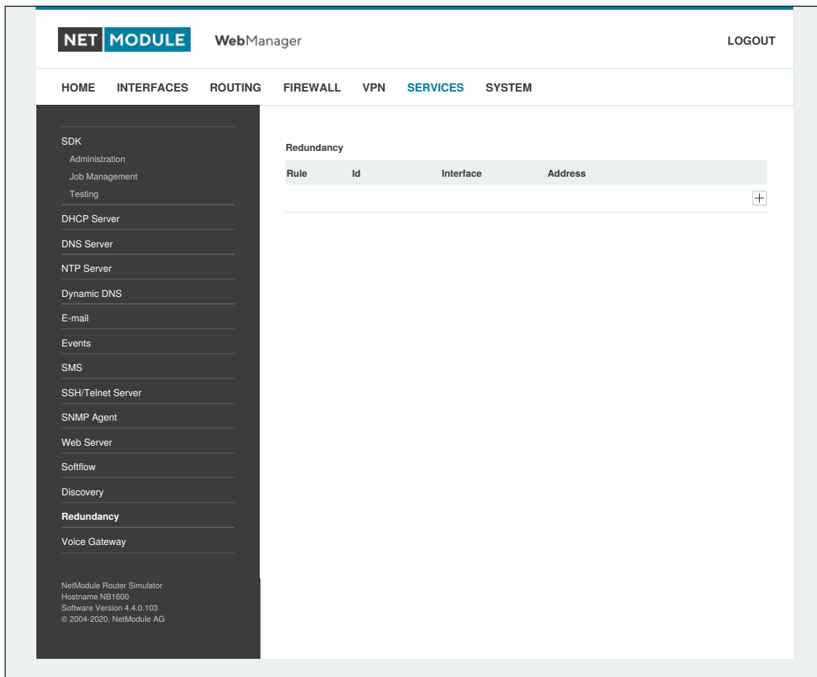
Abbildung 6.51.: VRRP-Konfiguration
