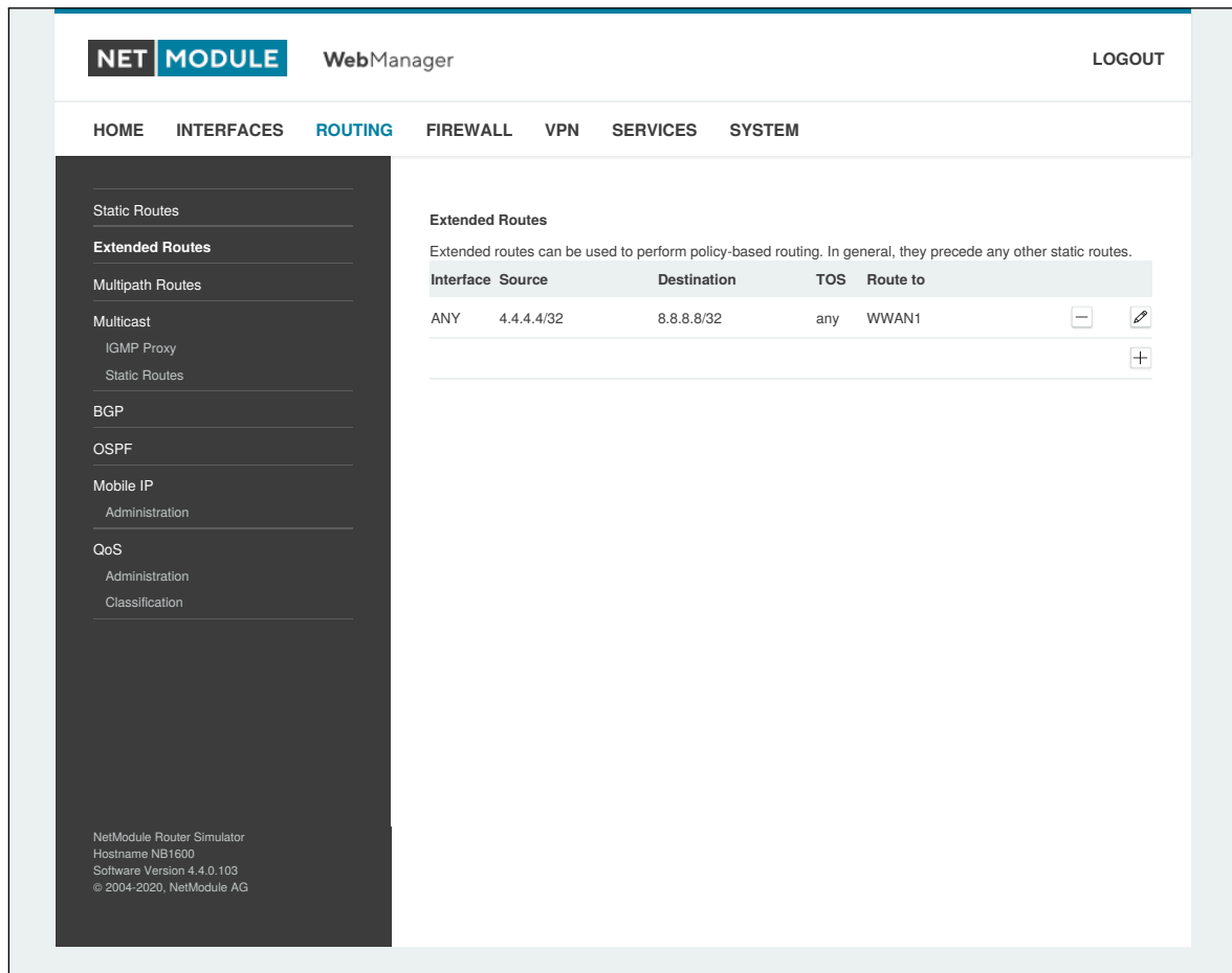
Abbildung 6.24.: Erweitertes Routing
