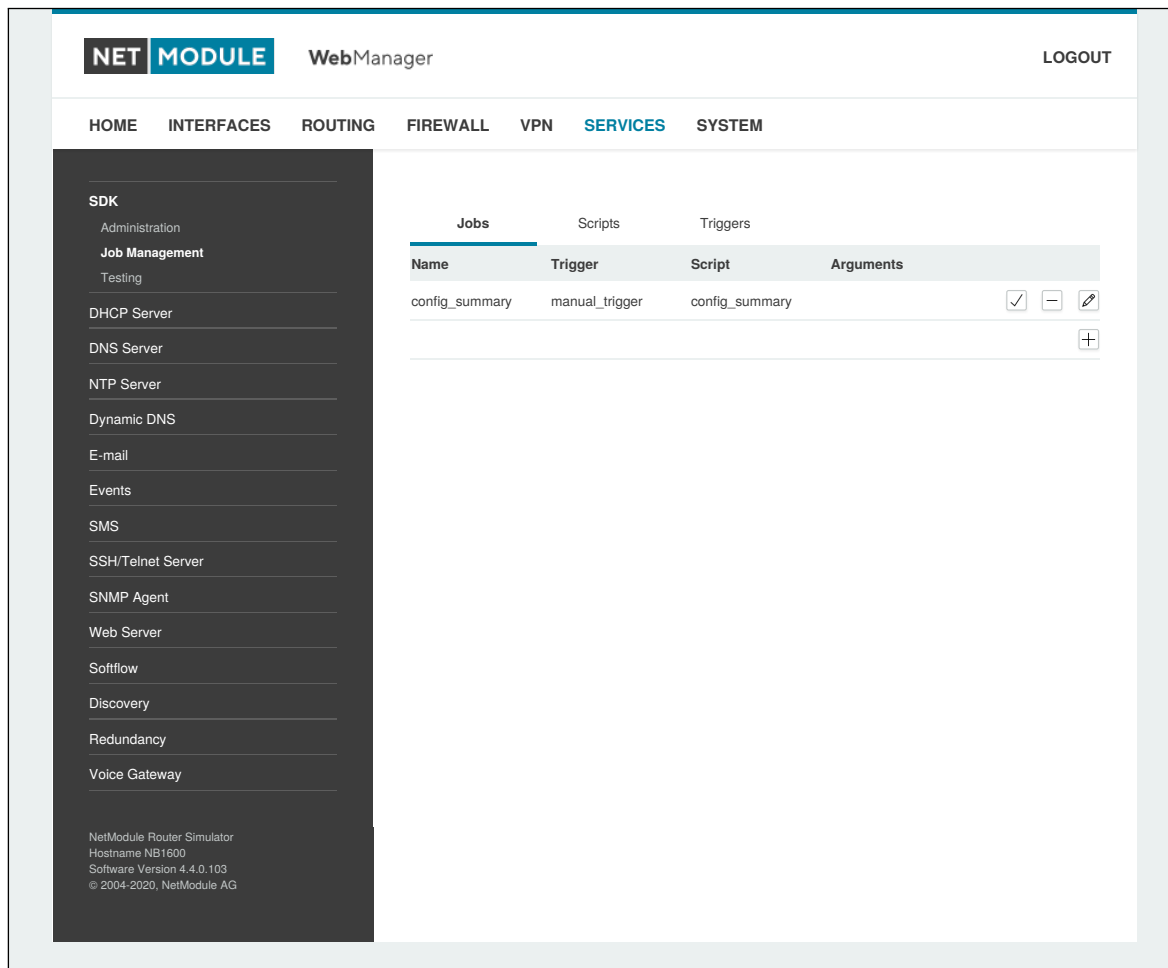
Abbildung 6.41.: SDK-Jobs
