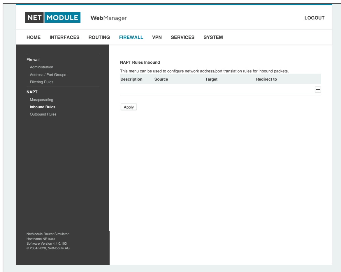
Abbildung 6.30.: NAPT-Regeln für eingehende Pakete
