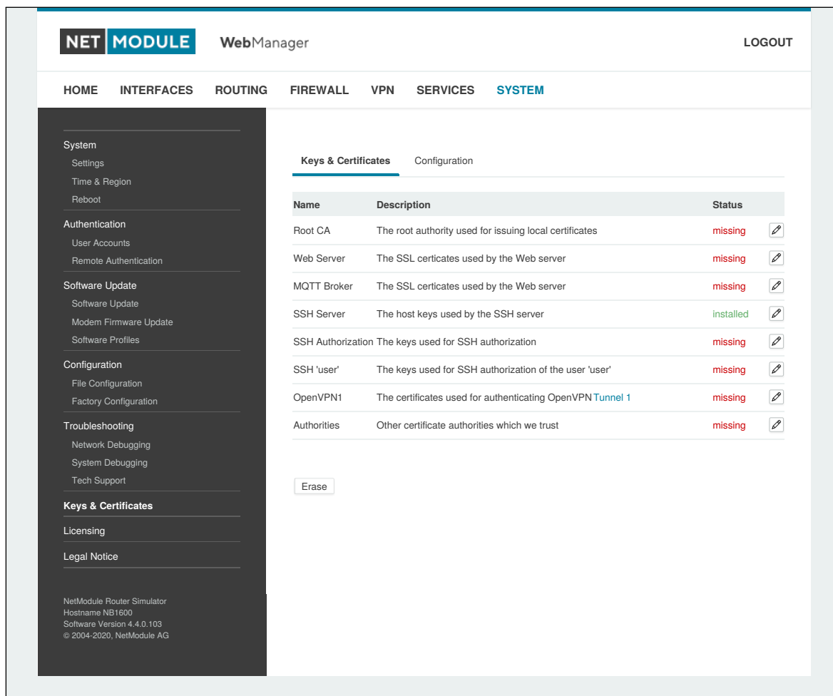
Abbildung 6.73.: Schlüssel und Zertifikate
