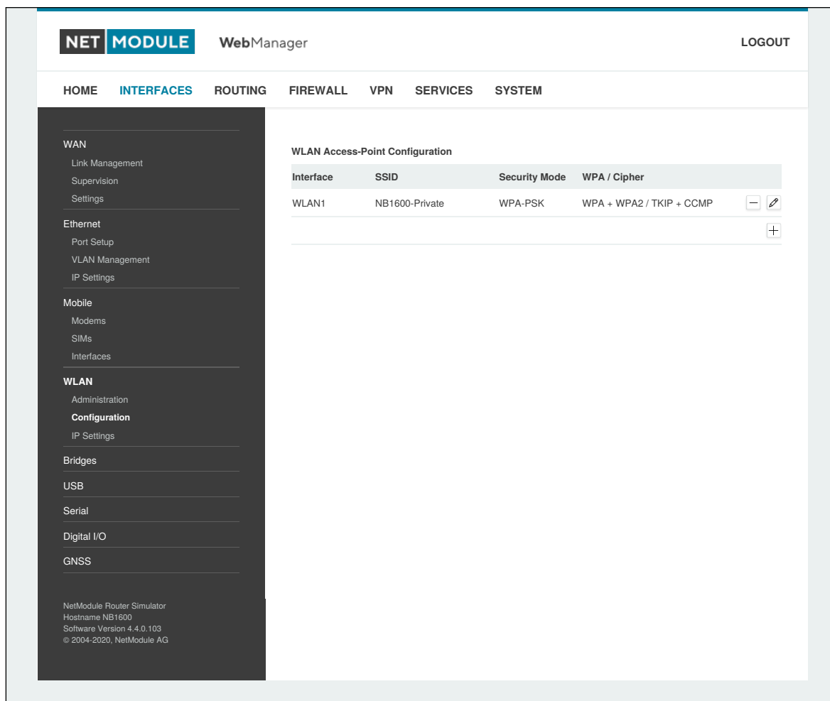
Abbildung 6.63.: WLAN administration
