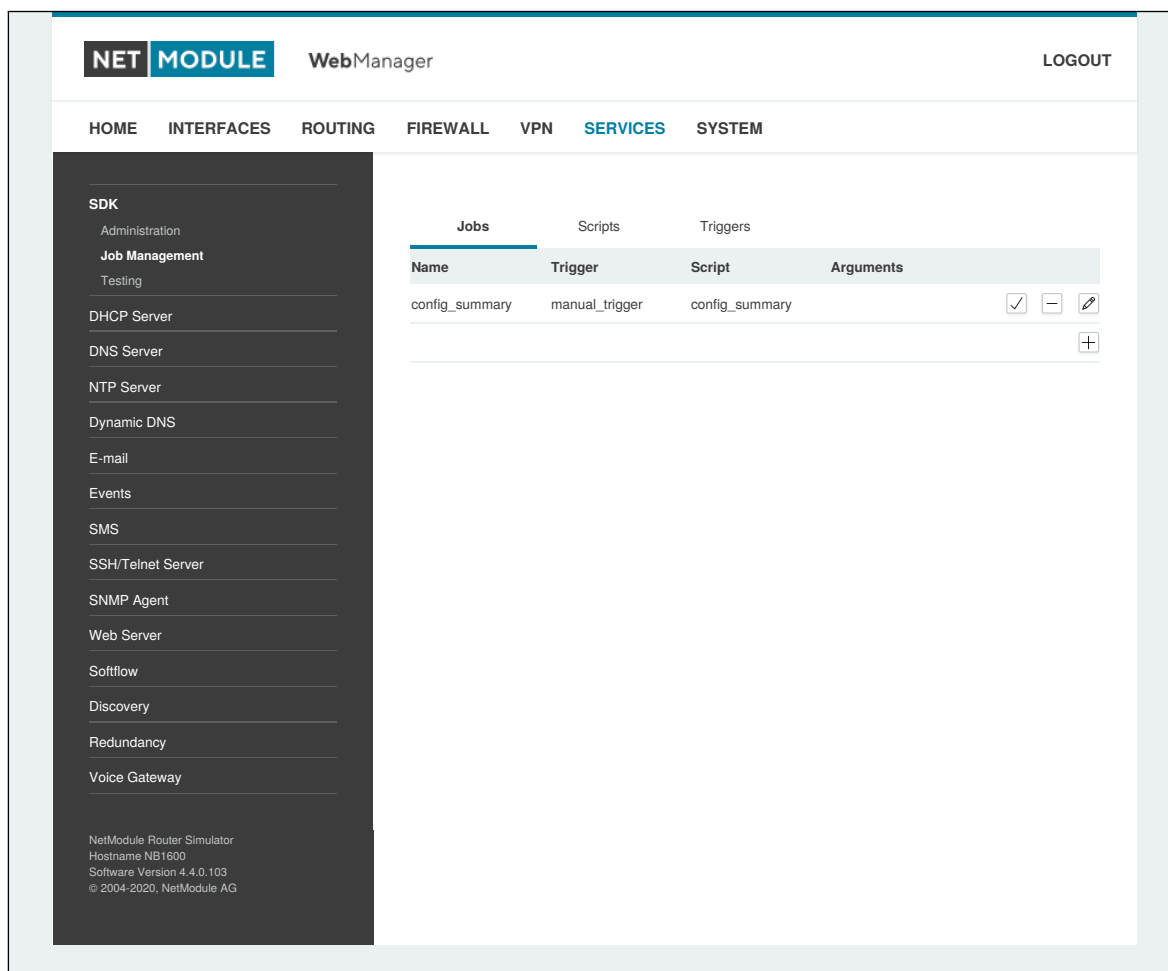
Abbildung 6.41.: SDK-Jobs
