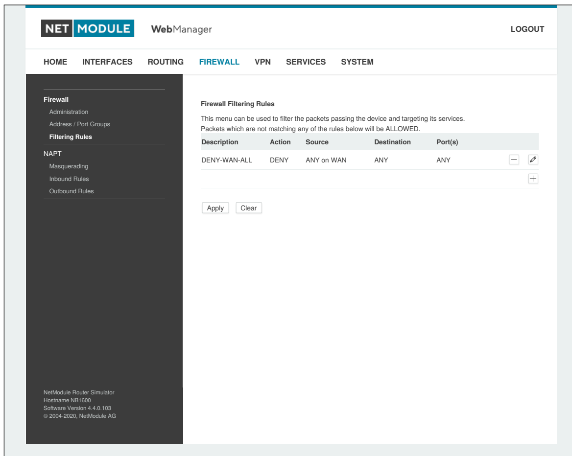
Abbildung 6.29.: Firewall-Regeln
