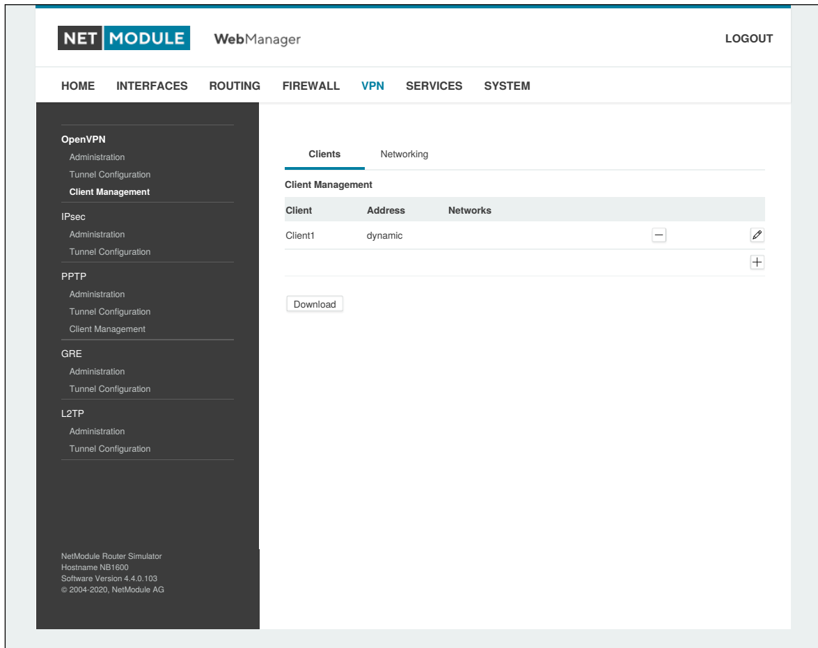
Abbildung 6.34.: OpenVPN-Client-Verwaltung
