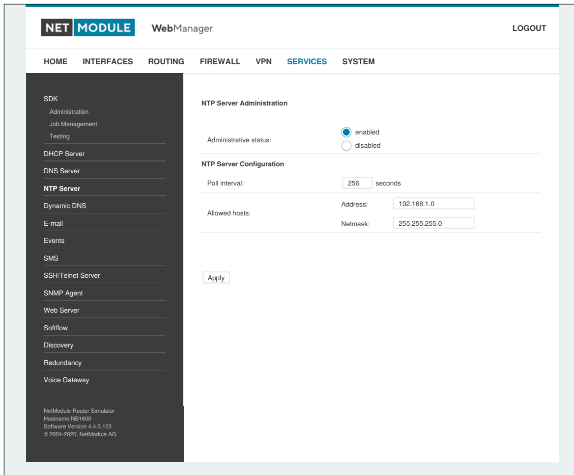
Abbildung 6.46.: NTP-Server
