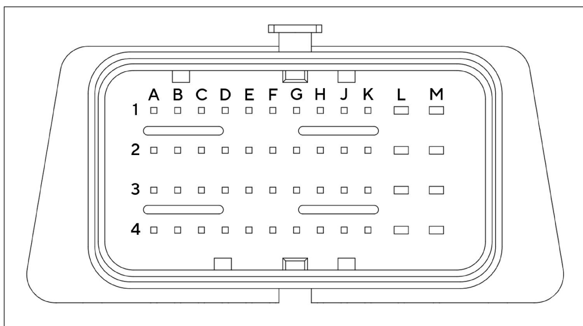
Abbildung 4.4.: X48 Outline
