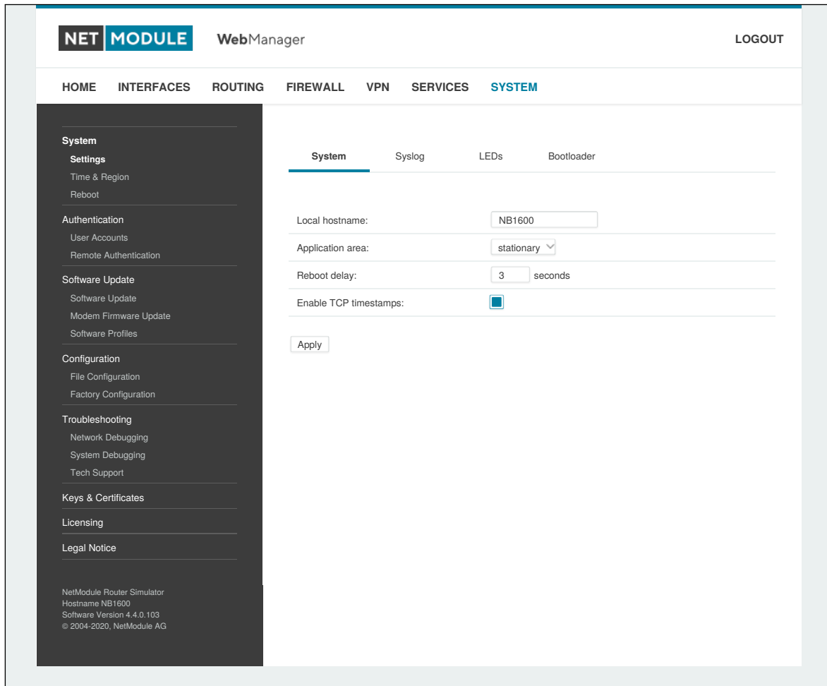
Abbildung 6.65.: System
