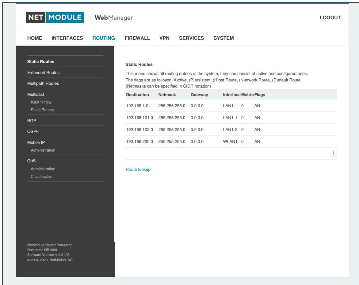
Abbildung 6.24.: Statisches Routing
