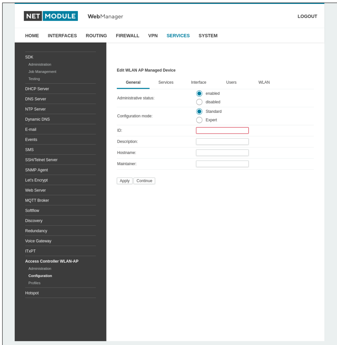
Abbildung 6.59.: AC WLAN-AP Configuration
