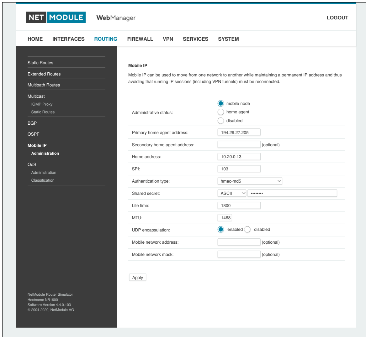
Abbildung 6.26.: Mobile IP
