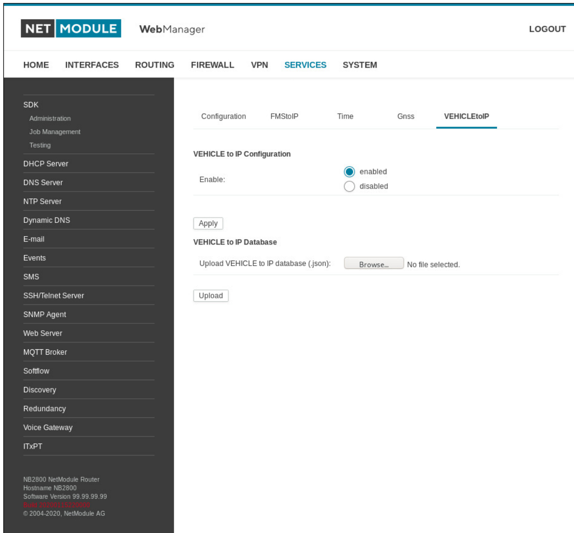
Abbildung 6.56.: ITxPT VEHICLEtoIP
