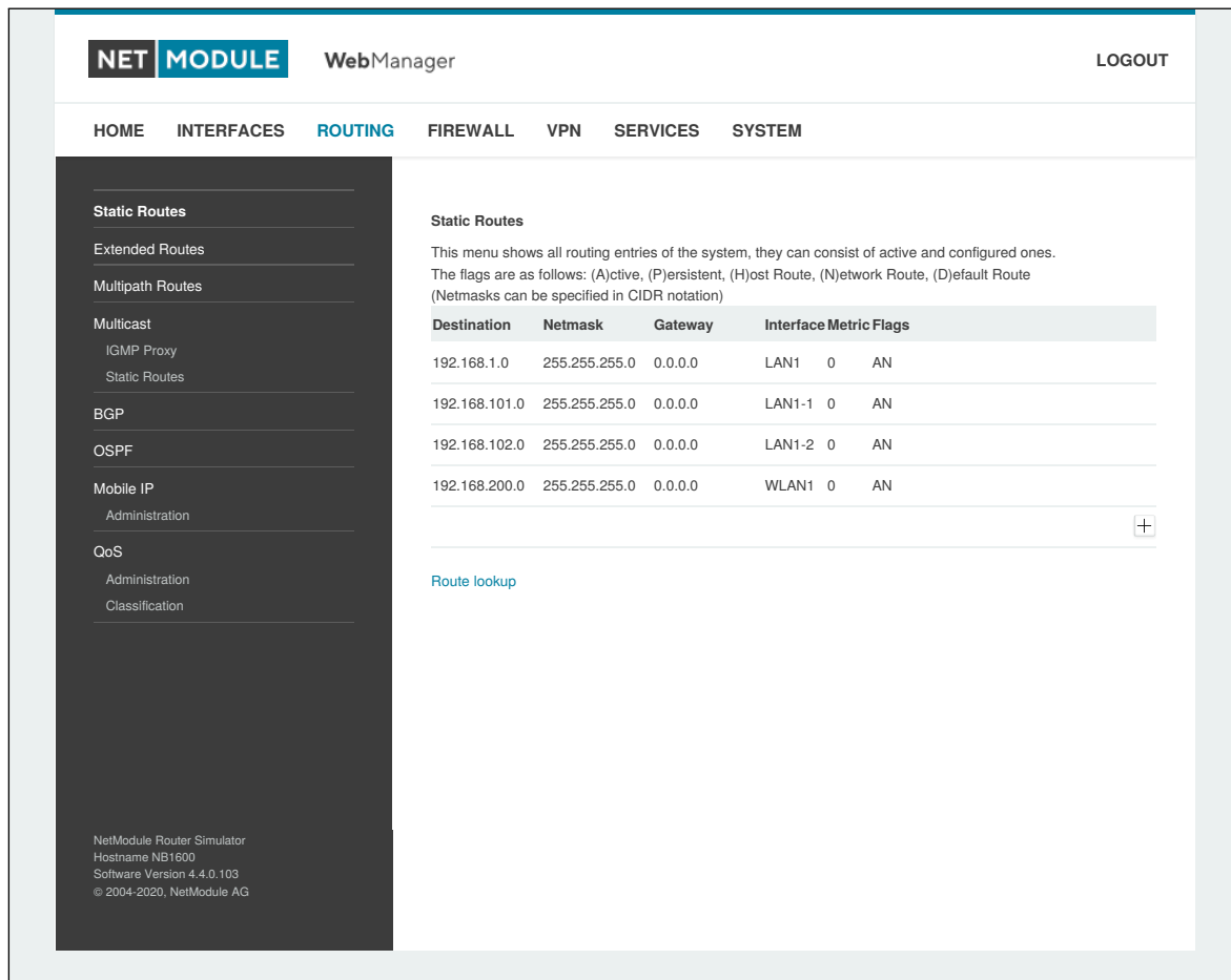
Abbildung 6.23.: Statisches Routing
