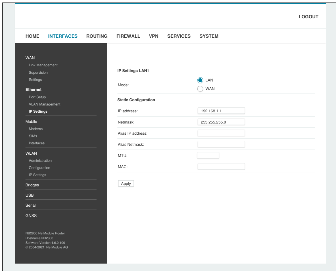
Abbildung 6.12.: IP Einstellungen - LAN Schnittstelle
