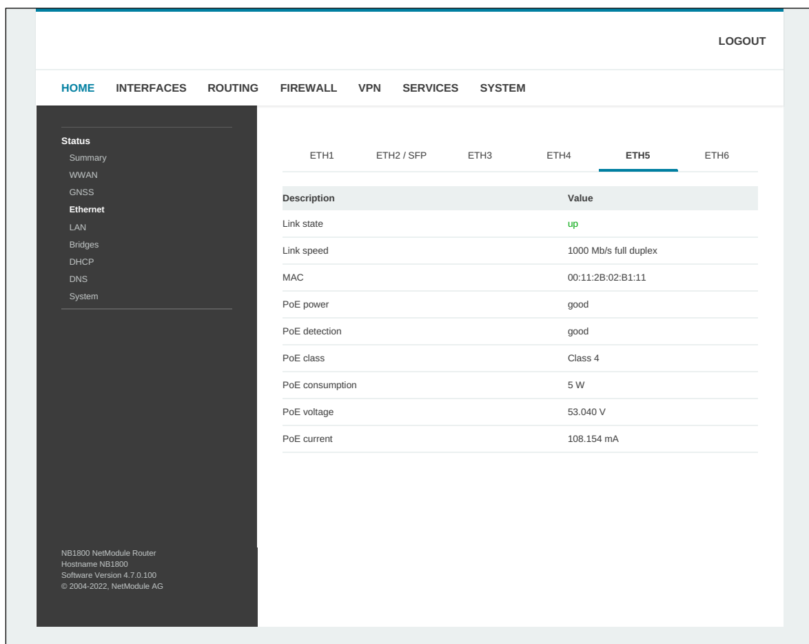
Abbildung 6.2.: Status des PoE-Power-Supply
