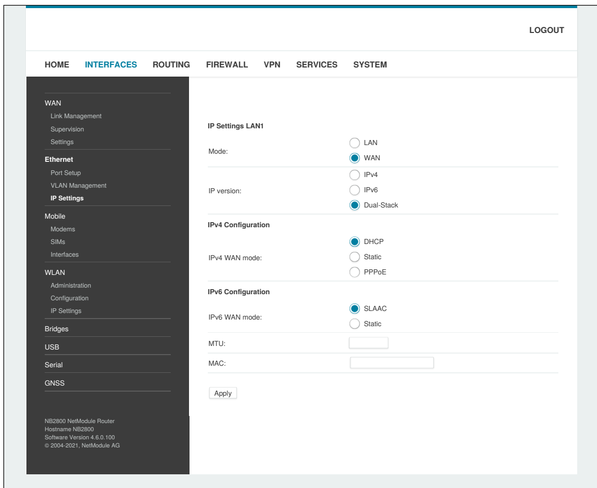
Abbildung 6.13.: IP Einstellungen - WAN Schnittstelle
