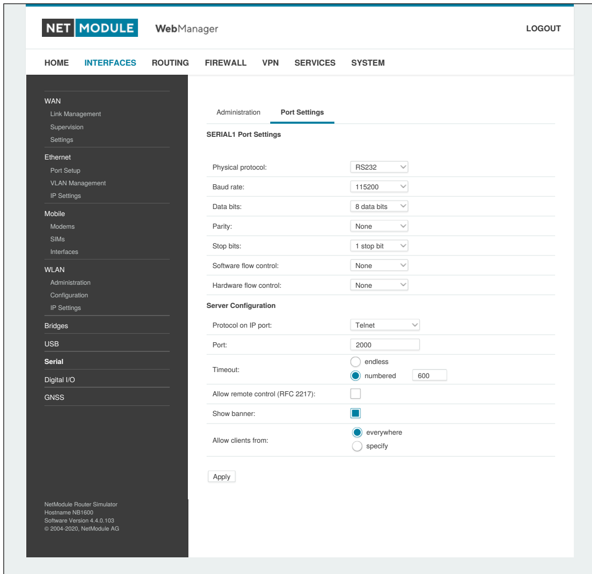
Abbildung 6.24.: Einstellungen der seriellen Schnittstelle
