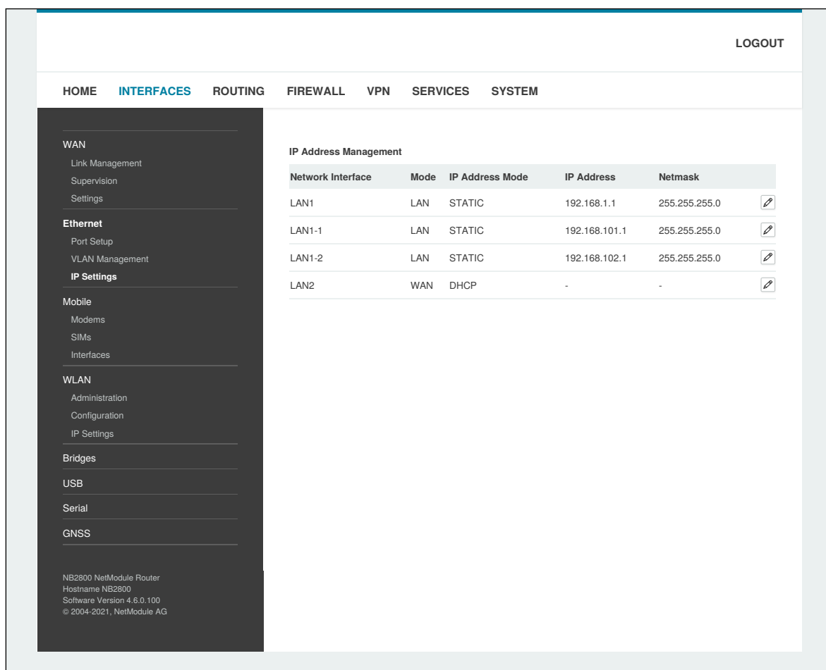
Abbildung 6.11.: IP Einstellungen - Übersicht
