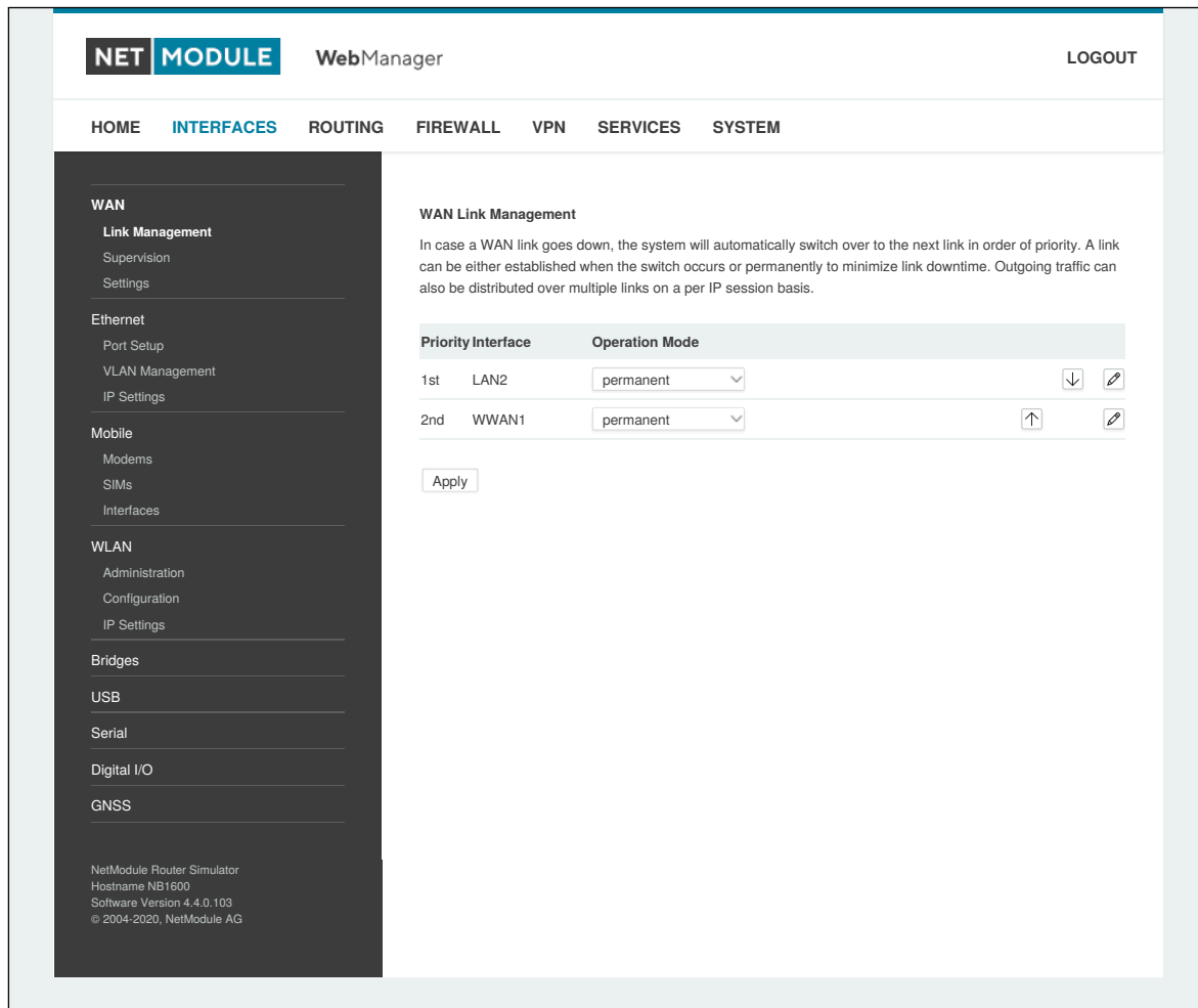
Abbildung 6.2.: WAN-Verbindungen
