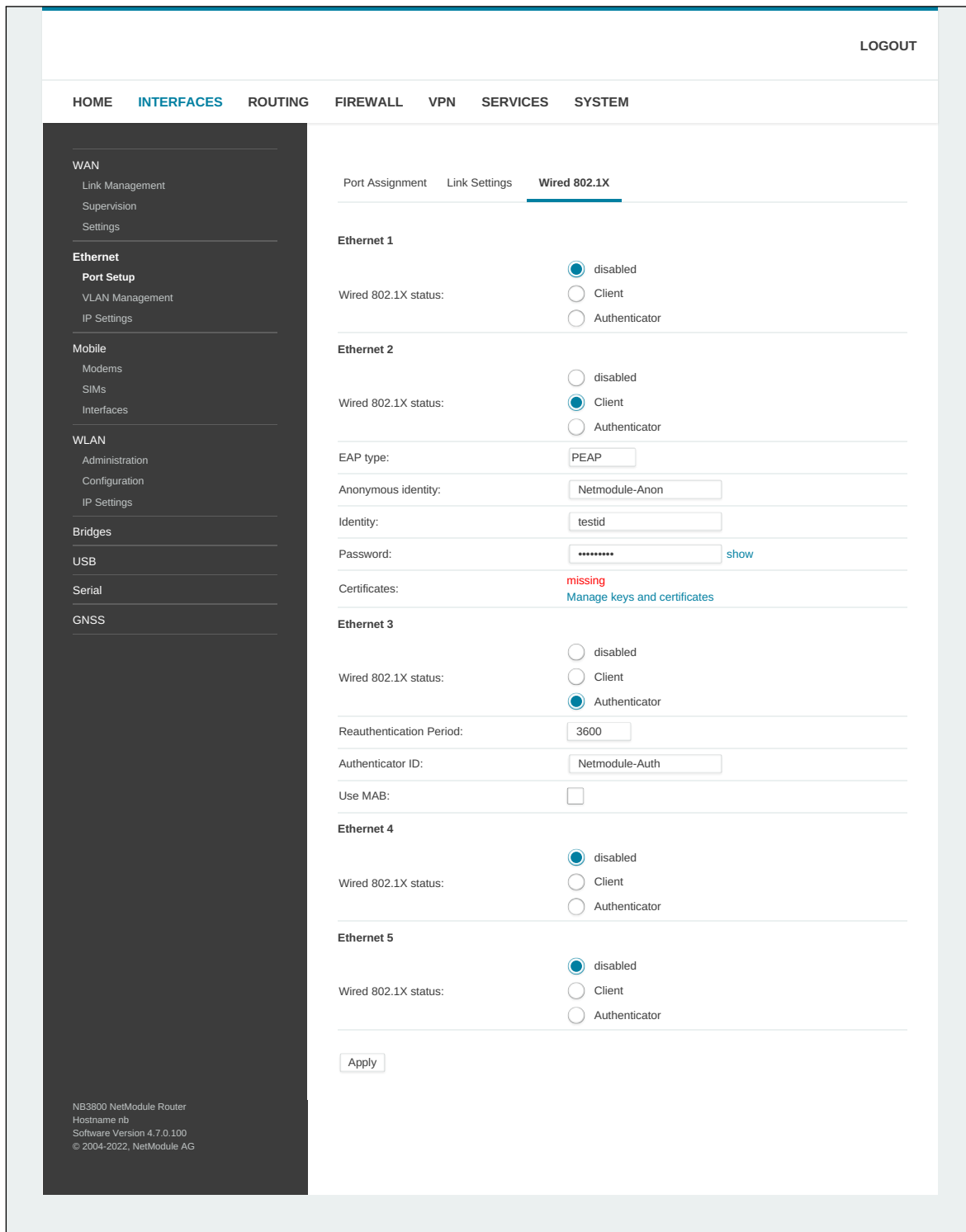
Abbildung 6.7.: Authentifizierung nach IEEE 802.1X
