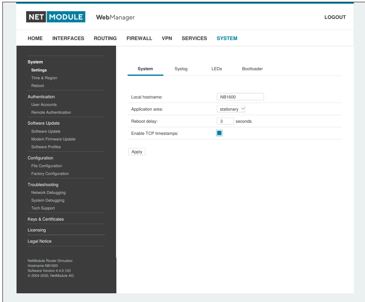
Abbildung 6.64.: System
