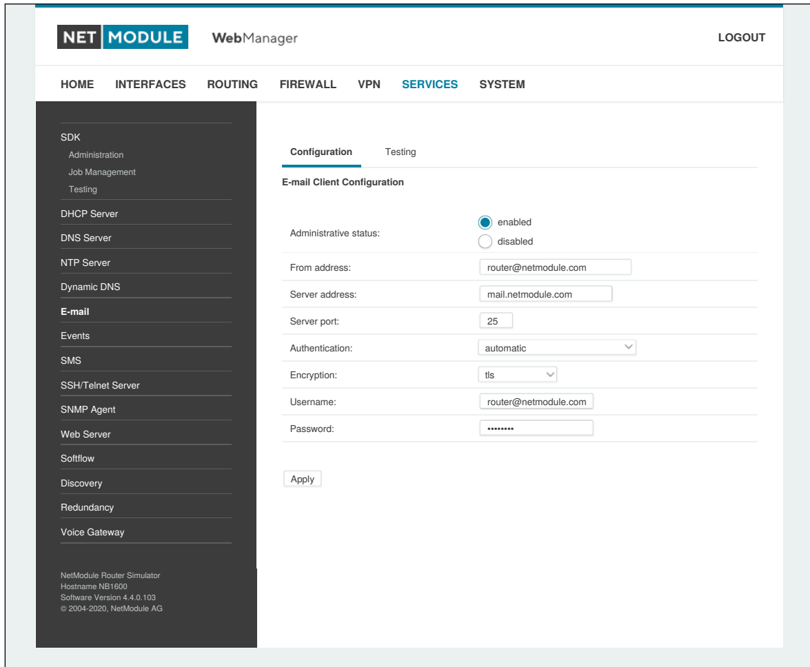
Abbildung 6.46.: E-Mail-Einstellungen
