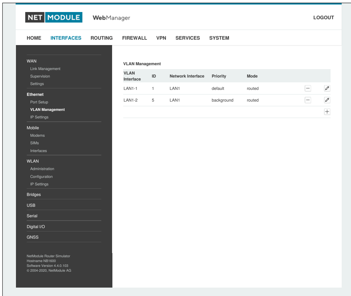
Abbildung 6.8.: VLAN-Verwaltung
