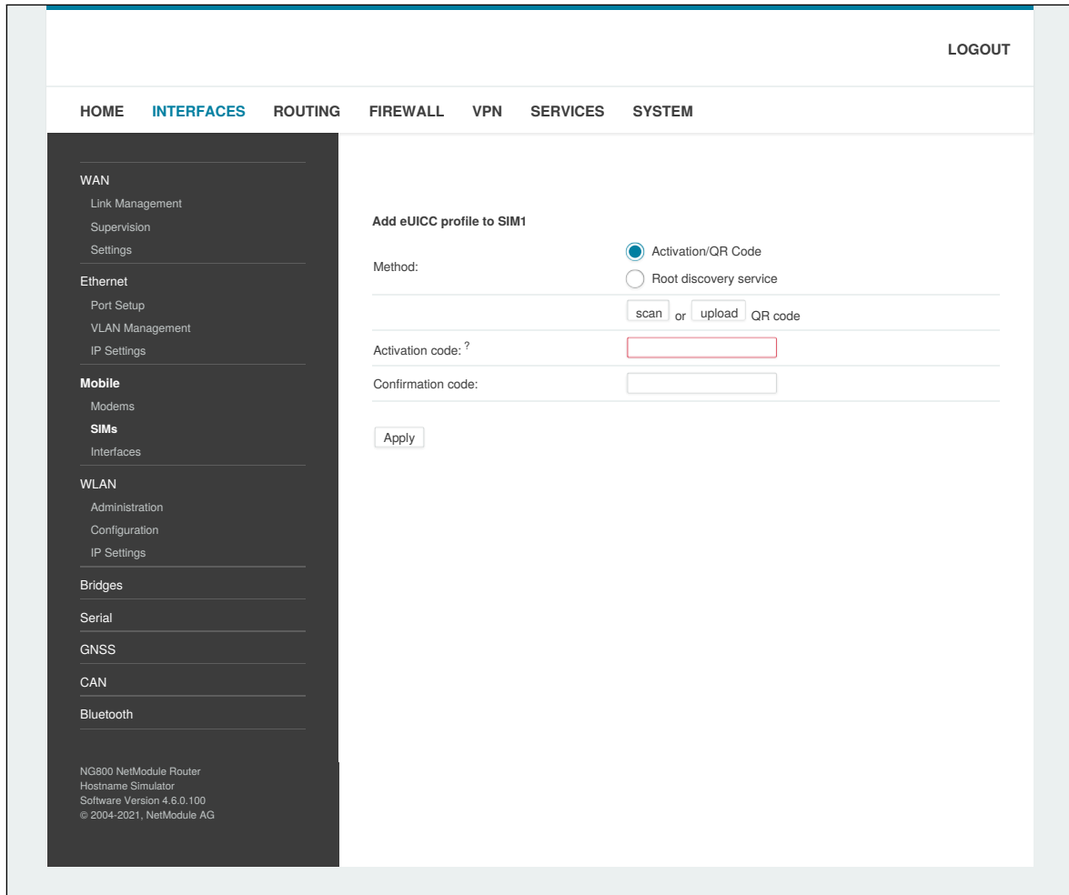
Abbildung 6.14.: eUICC-Profil hinzufügen
