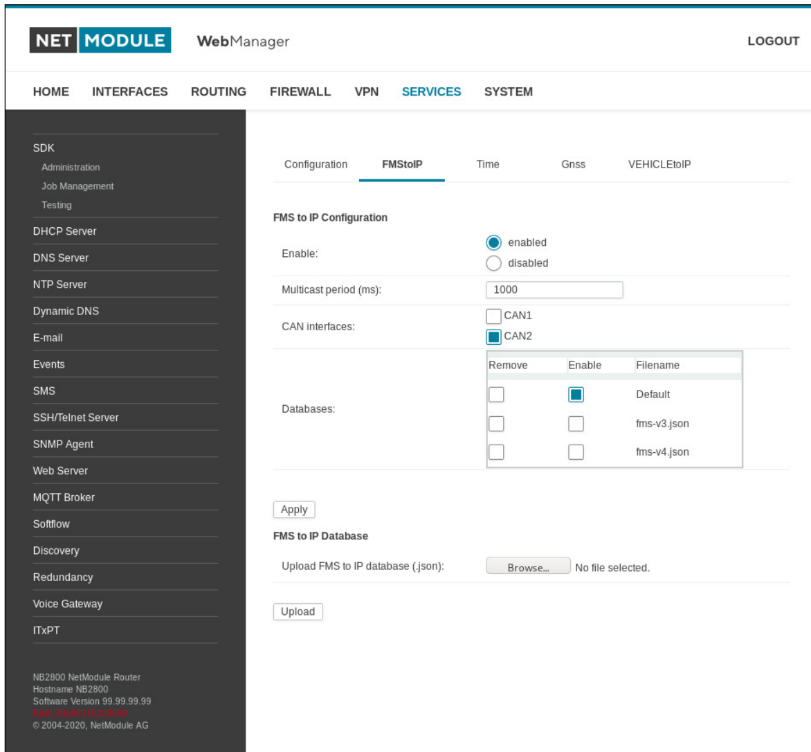
Abbildung 6.53.: ITxPT FMS-to-IP
