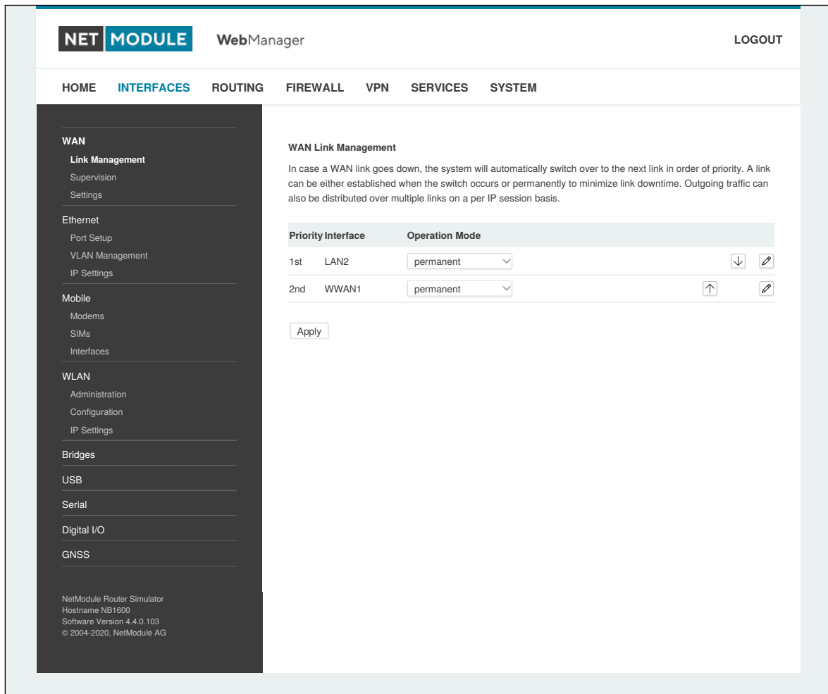
Abbildung 6.2.: WAN-Verbindungen
