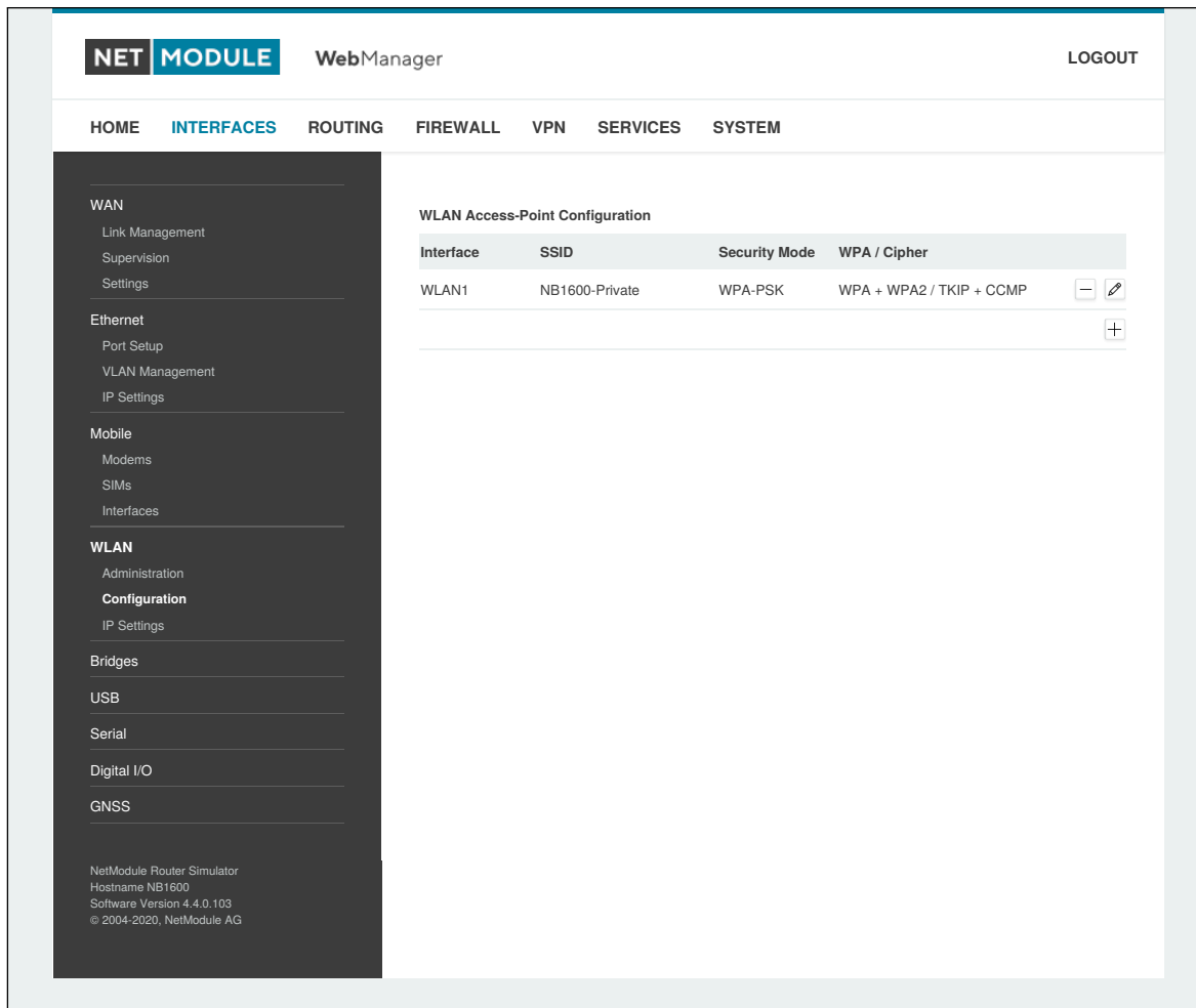
Abbildung 6.63.: WLAN administration
