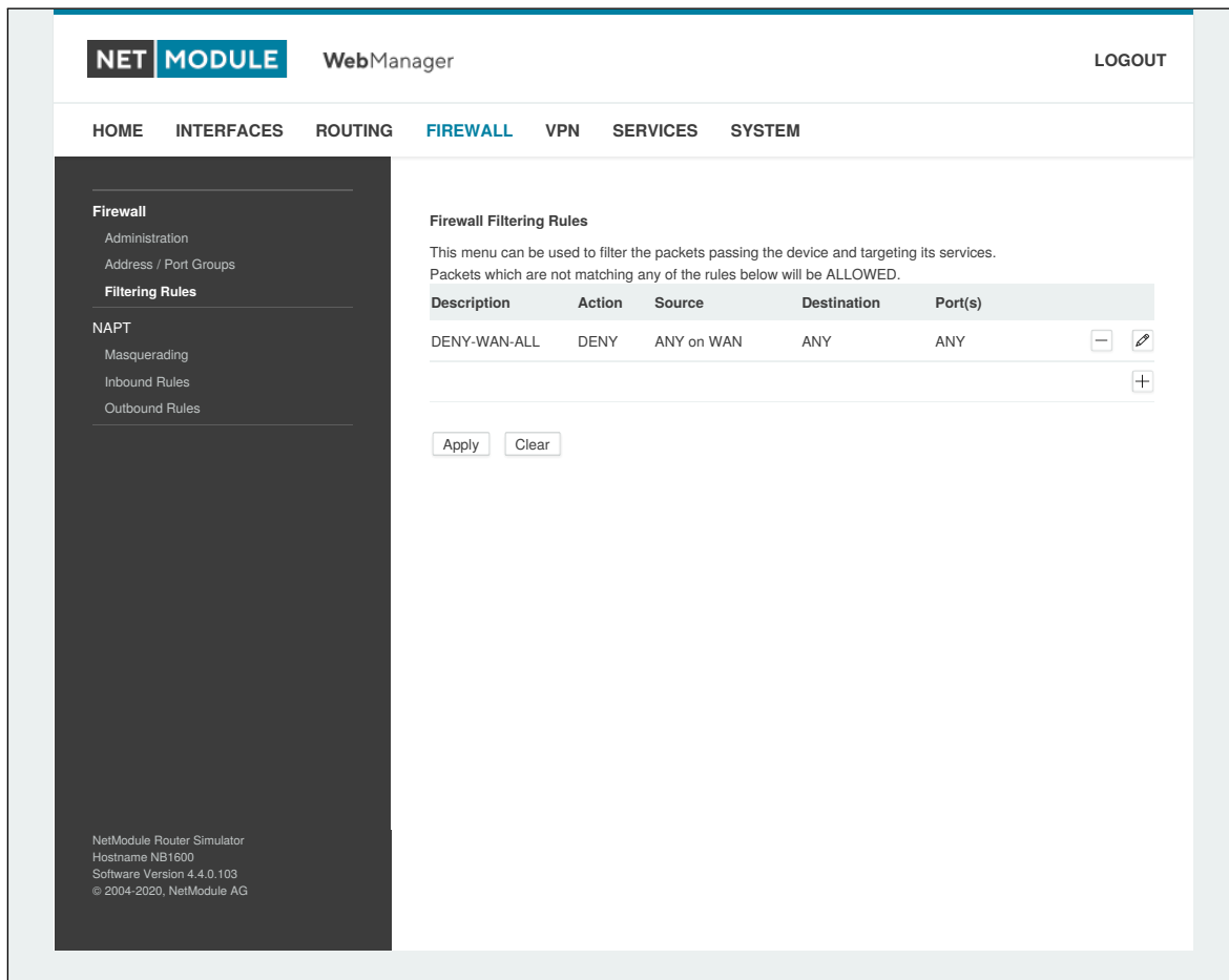
Abbildung 6.28.: Firewall-Regeln
