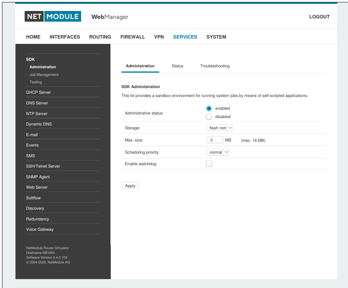
Abbildung 6.40.: SDK-Verwaltung
