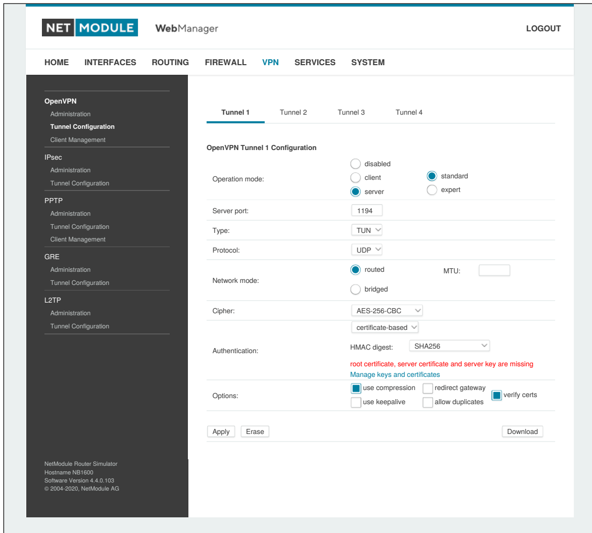
Abbildung 6.32.: Konfiguration von OpenVPN
