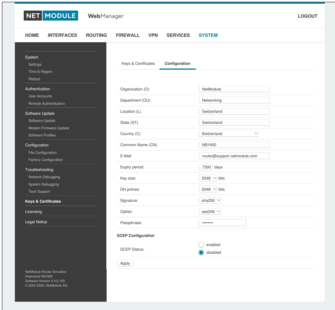
Abbildung 6.74.: Konfiguration von Zertifikaten
