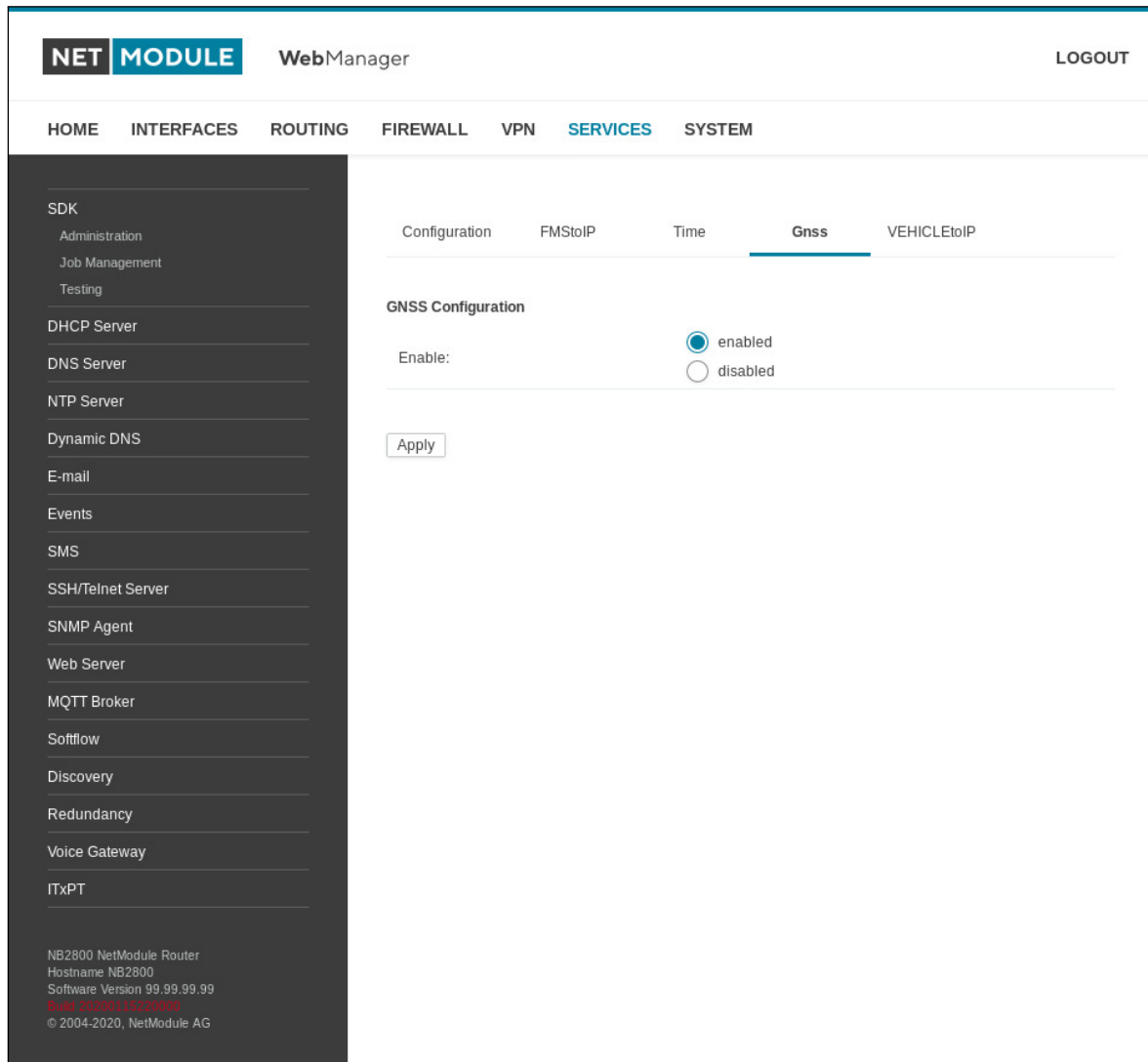
Abbildung 6.54.: ITxPT GNSS
