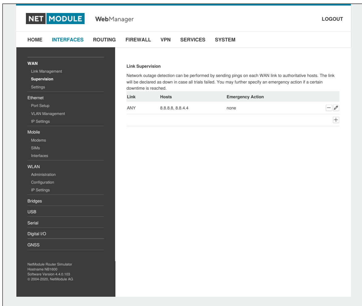
Abbildung 6.3.: Verbindungsüberwachung
