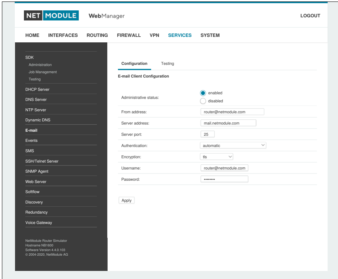
Abbildung 6.46.: E-Mail-Einstellungen
