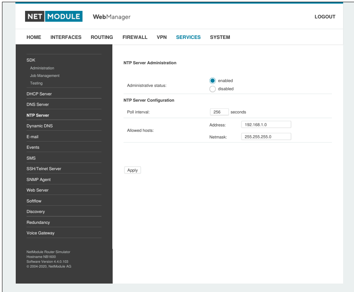
Abbildung 6.44.: NTP-Server
