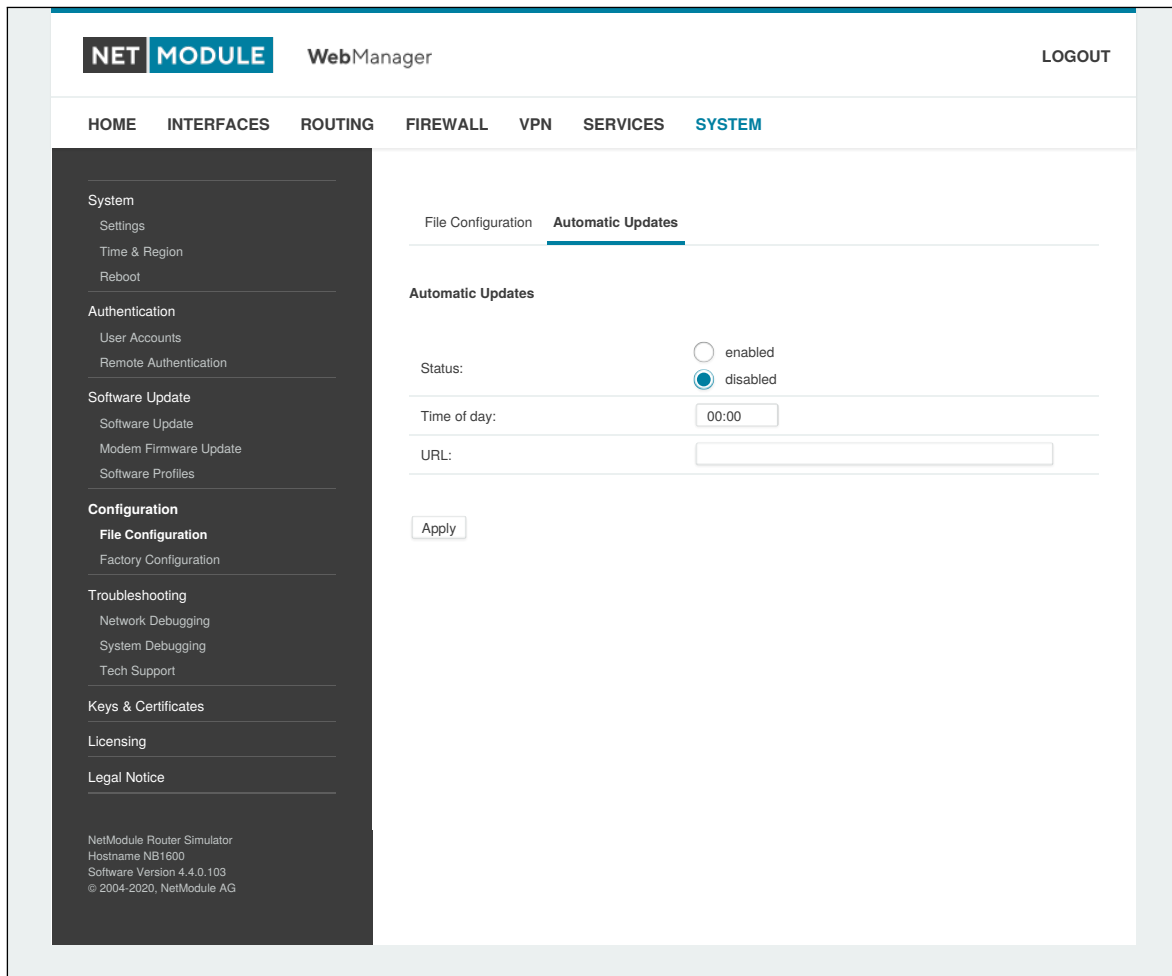
Abbildung 6.69.: Automatische Konfiguration per Datei
