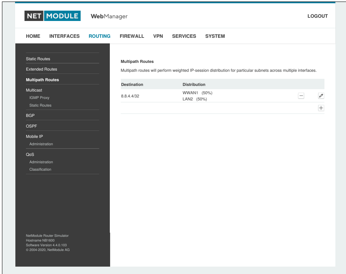
Abbildung 6.25.: Multipath-Routing
