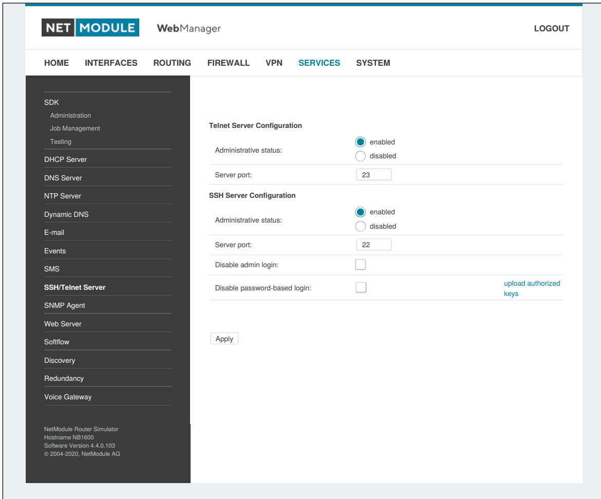
Abbildung 6.48.: SSH- und Telnet-Server
