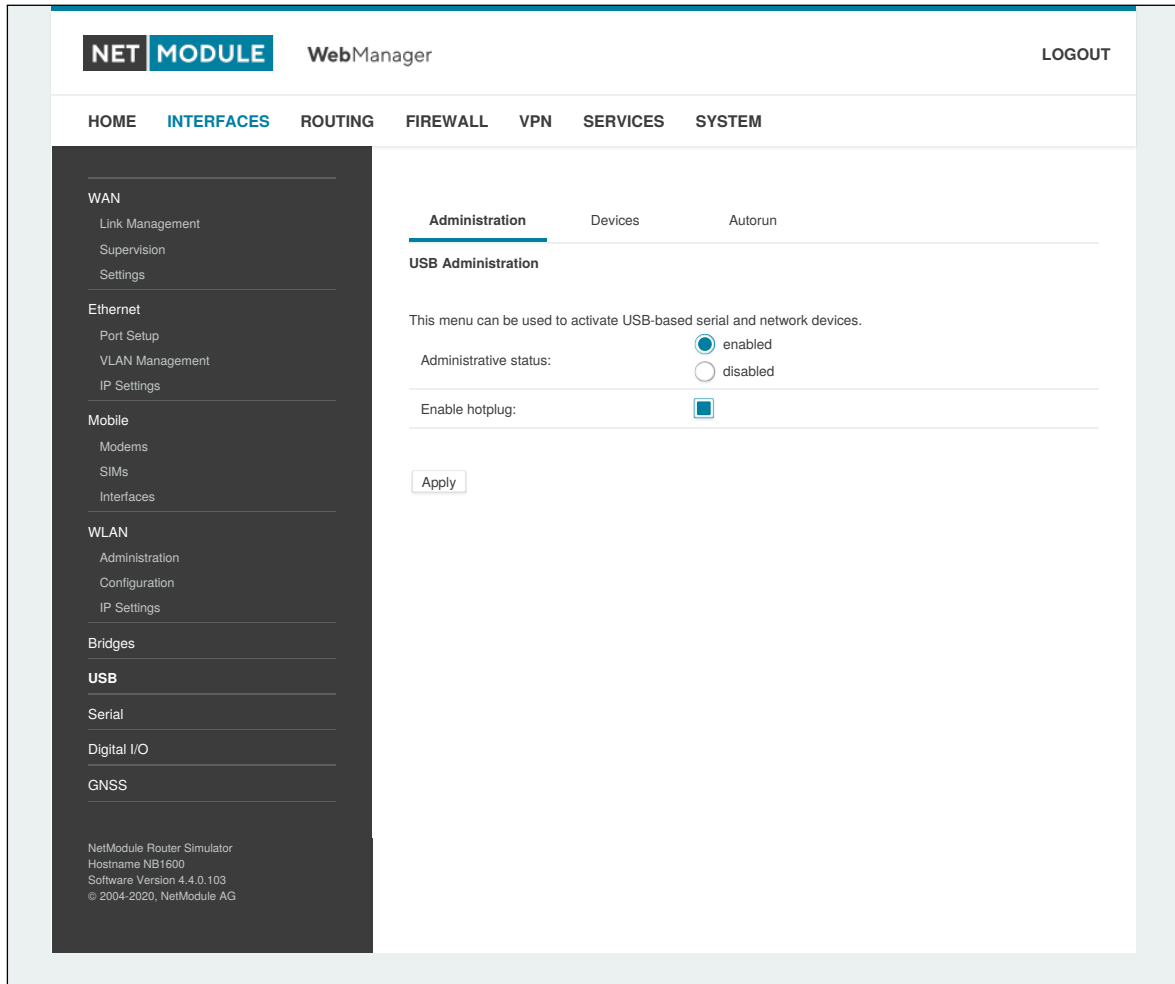
Abbildung 6.19.: USB-Verwaltung
