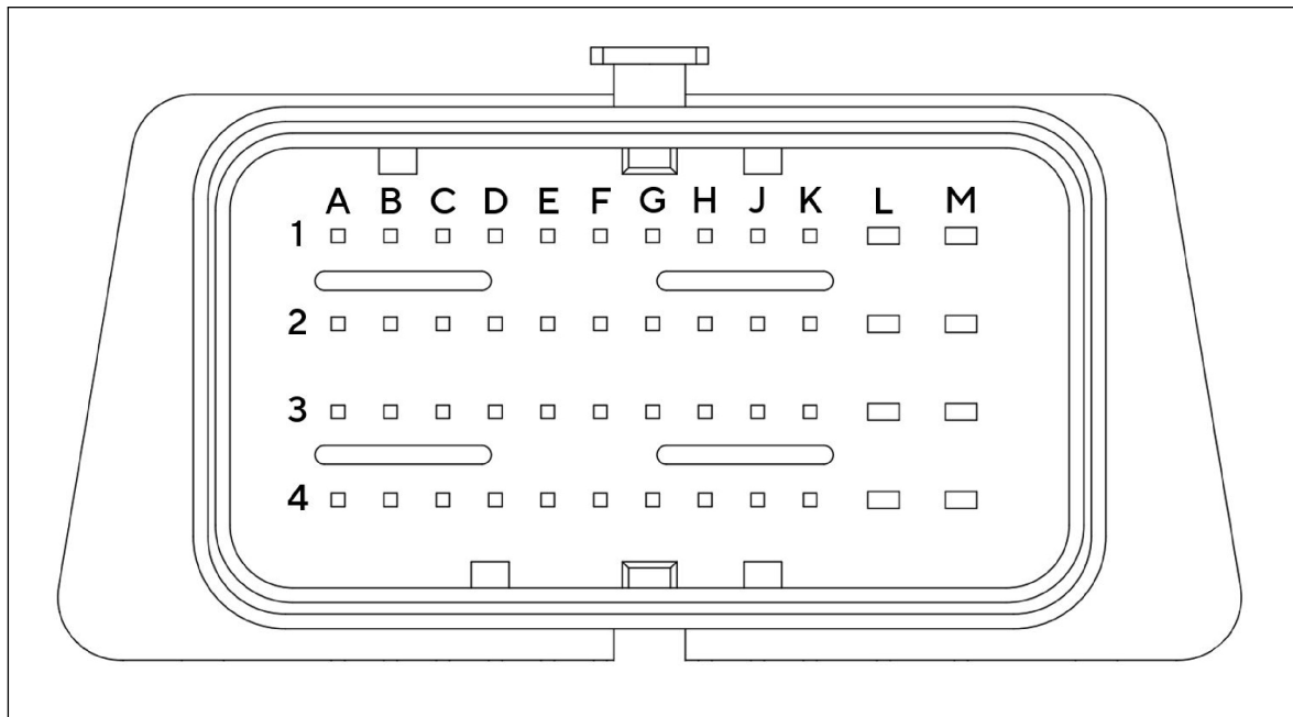
Abbildung 4.4.: X48 Outline
