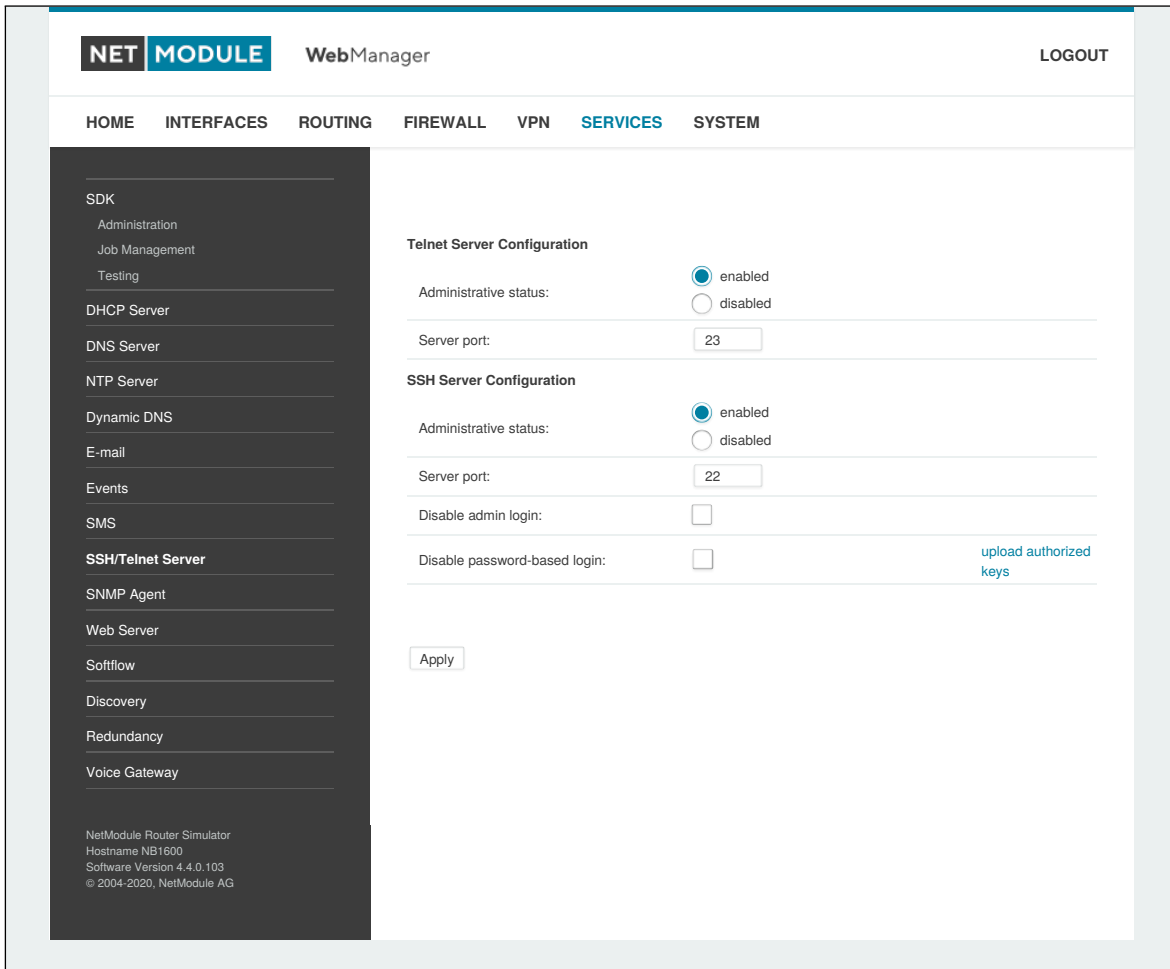
Abbildung 6.46.: SSH- und Telnet-Server
