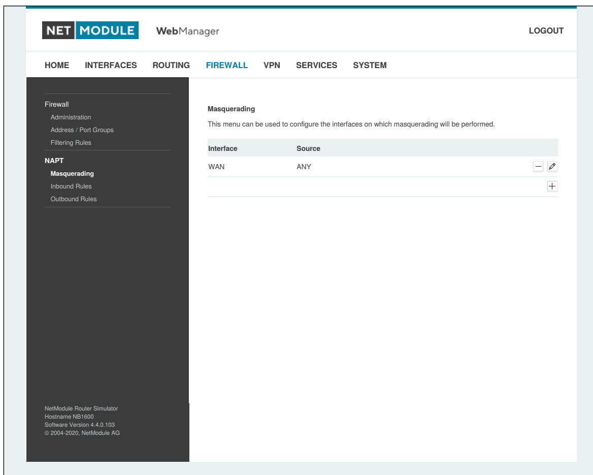
Abbildung 5.25.: Maskierung (Masquerading)
