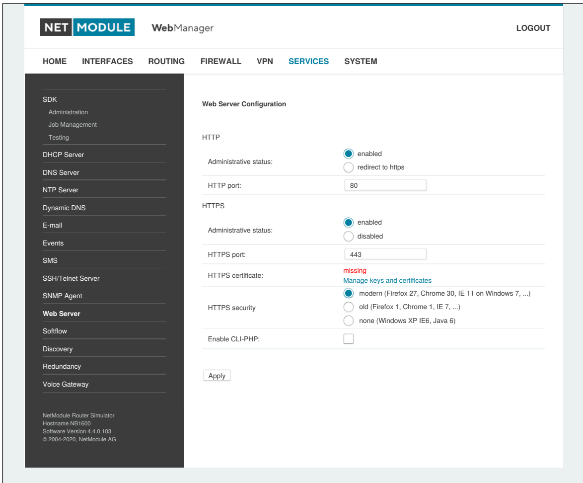
Abbildung 5.46.: Webserver
