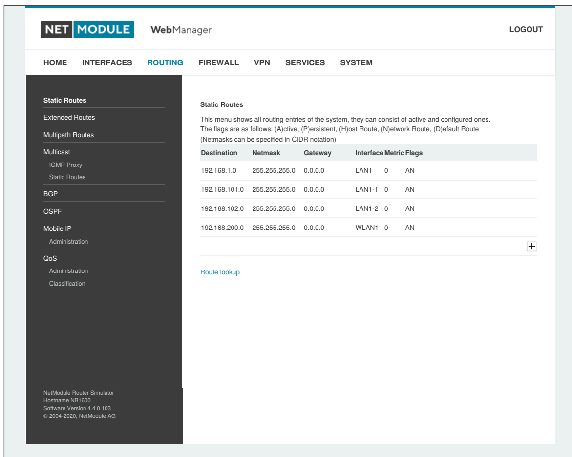
Abbildung 5.19.: Statisches Routing
