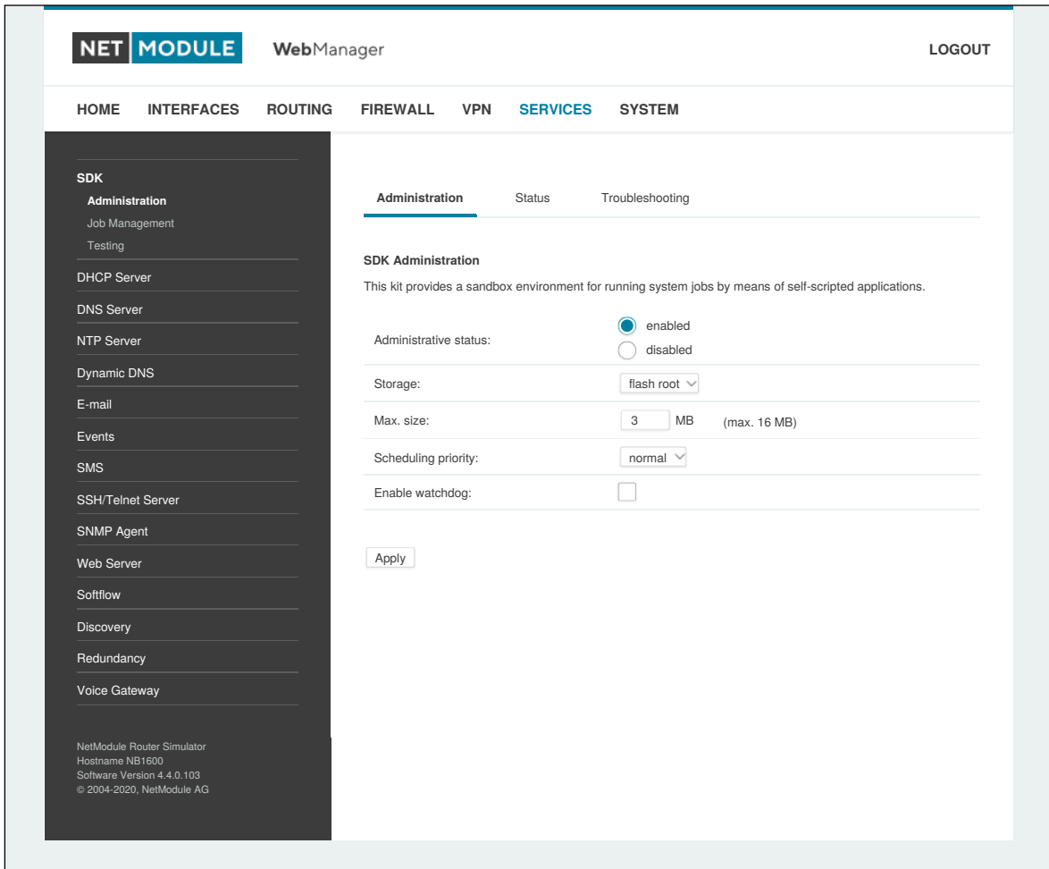
Abbildung 5.37.: SDK-Verwaltung
