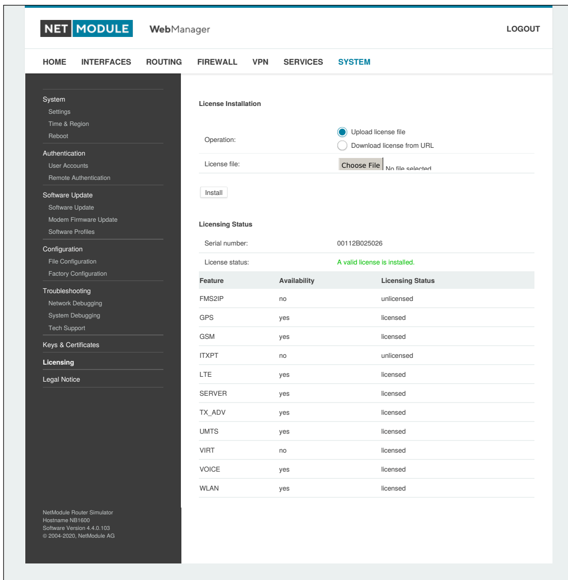
Abbildung 5.61.: Lizenzierung
