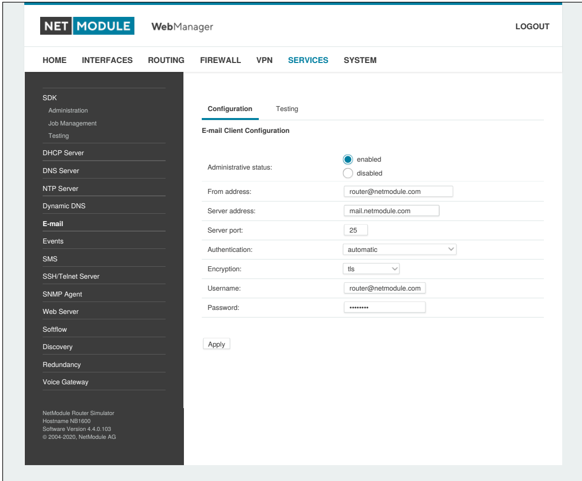
Abbildung 5.43.: E-Mail-Einstellungen
