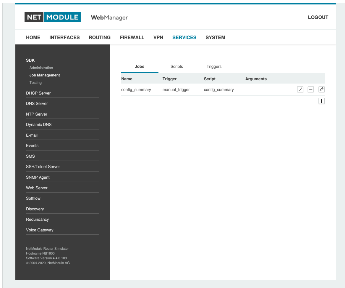
Abbildung 5.37.: SDK-Jobs
