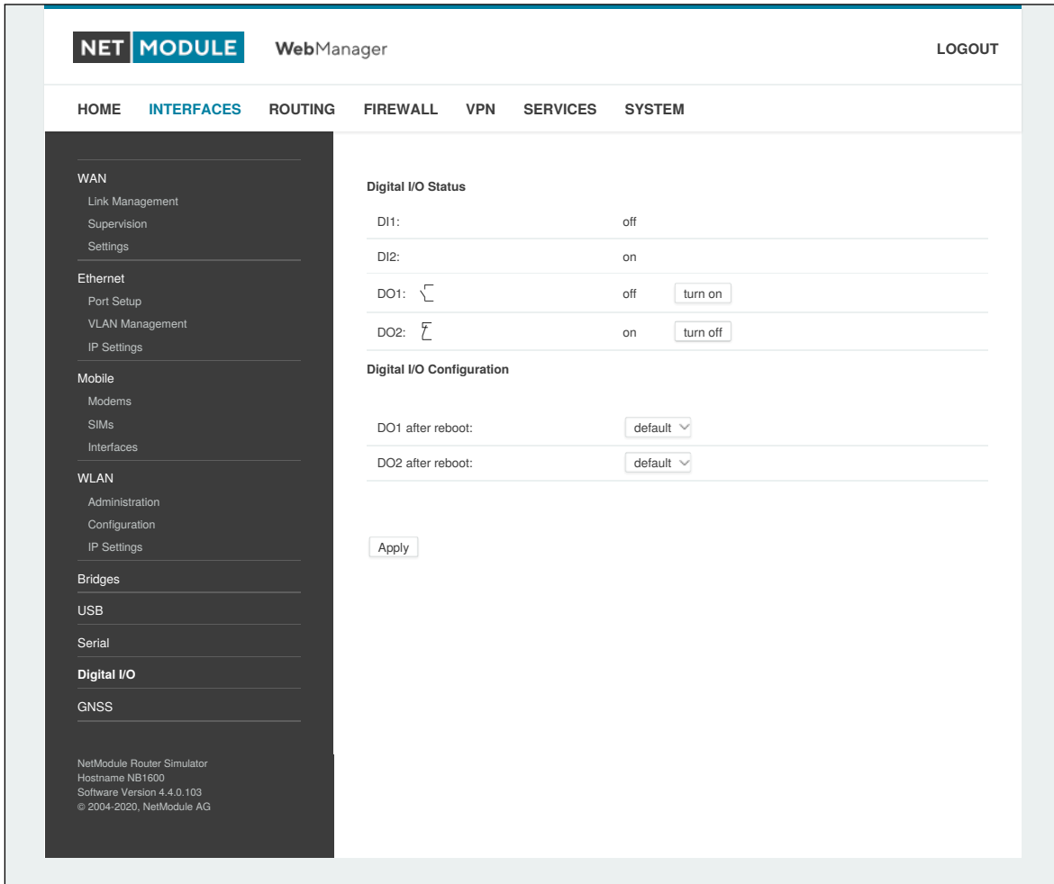
Abbildung 5.19.: Digitale Ein-/Ausgänge
