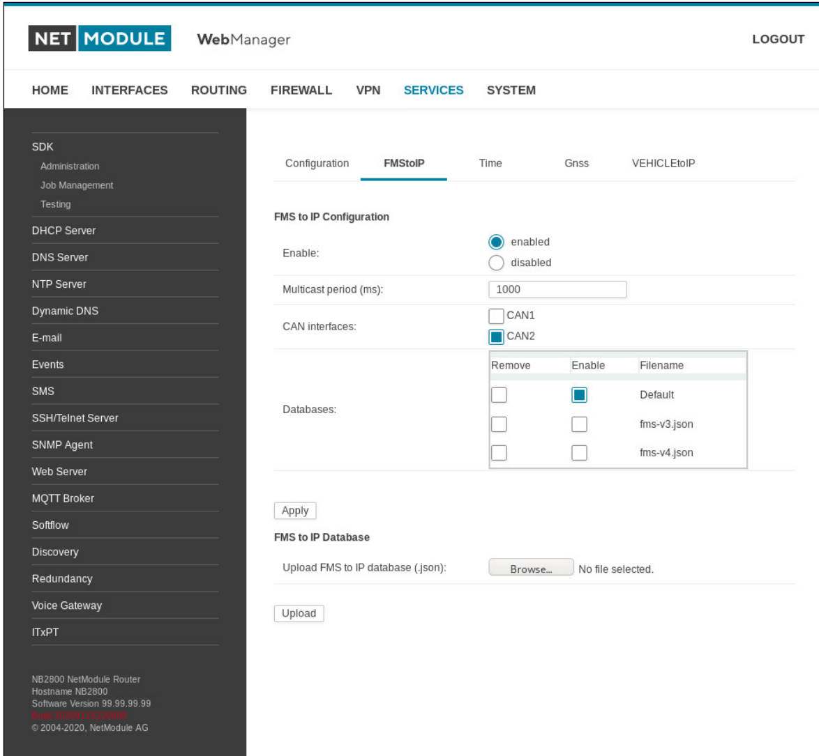
Abbildung 5.49.: ITxPT FMS-to-IP
